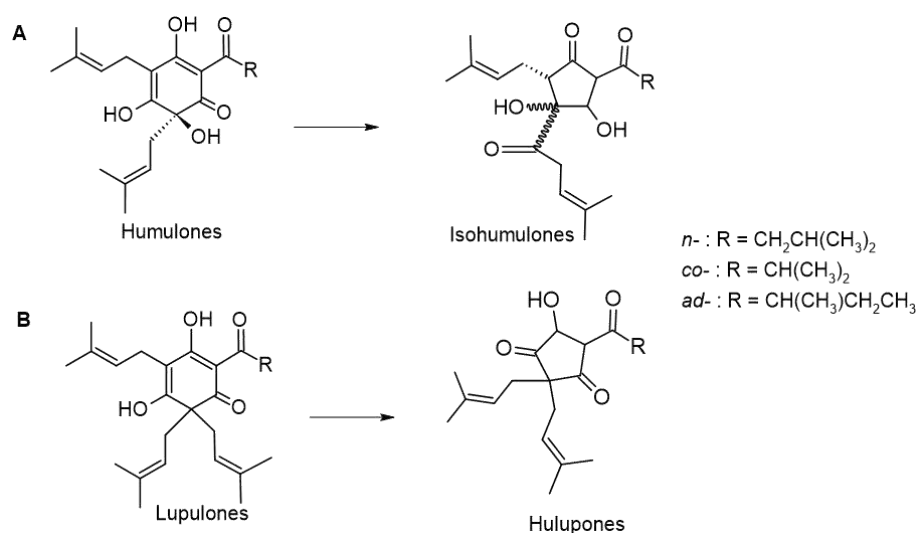
Figure 9. Transformation des acides \alpha (A) et \beta (B) au cours du processus de fabrication de la bière. L'isomérisation des acides \alpha en acides-iso- \alpha en position cis et trans .
