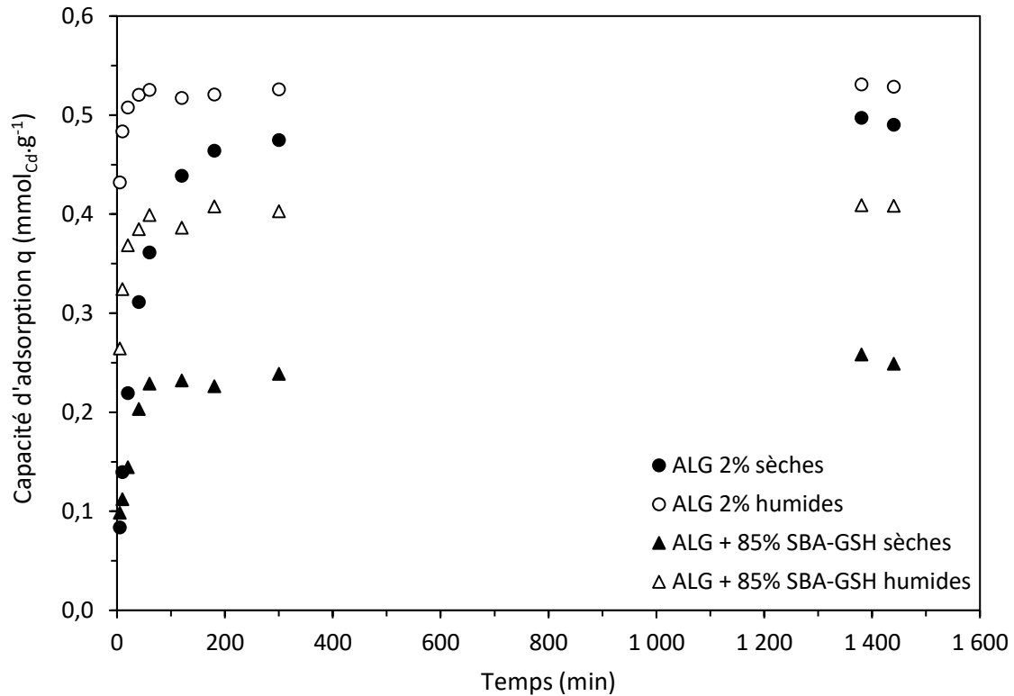
Figure 6.1 : Cinétiques d'adsorption de Cd(II) par des billes ALG 2% et ALG + 85% SBA-GSH humides et sèches ( C_0 = 8,0 \pm 0,5 \text{ mM}_{\text{Cd}} ; billes sèches ( 10 \text{ g} \cdot \text{L}^{-1} ) ou billes humides ( 10 \text{ g} \cdot \text{L}^{-1} équivalent billes sèches) ; étude mono-élémentaire ; milieu \text{NaNO}_3 0,1 \text{ M} ; agitation magnétique 500 \text{ rpm} ; 25 \pm 1^\circ \text{C} ; \text{pH} = 6,7 ). Erreur expérimentale : \leq 5\%
