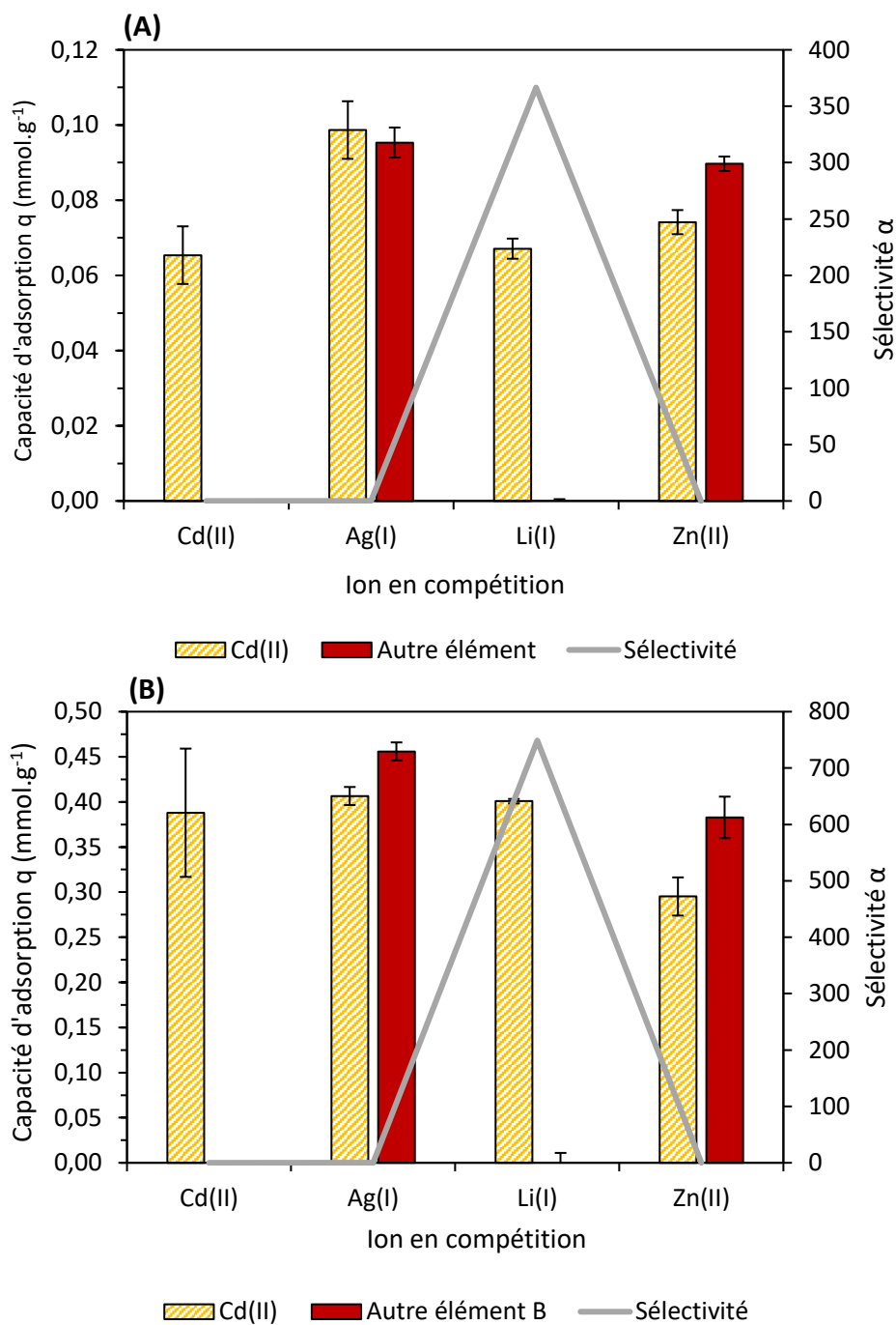
Figure 3 : Étude de la compétition entre Cd(II) et d'autres ions métalliques sur SBA-GSH à partir de solutions de concentration initiale 0,9 mM (A) ou 4,5 mM (B) par élément ( 10 \text{ g}\cdot\text{L}^{-1} de SBA-GSH ; agitation magnétique 500 rpm ; 25 \pm 1^\circ\text{C} ; 120 minutes de contact ; pH = 6,8)
