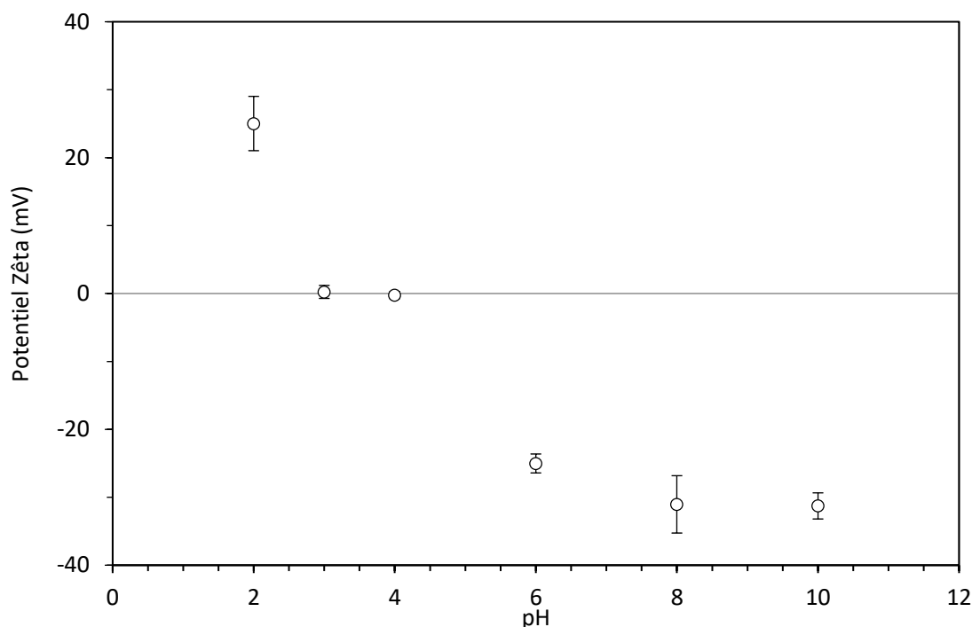
Figure 3.8 : Mesures du potentiel Zêta de SBA-GSH en fonction du pH (Milieu : H 2 O ; 0,005% massiques de SBA-GSH ; 25±0,1°C)
