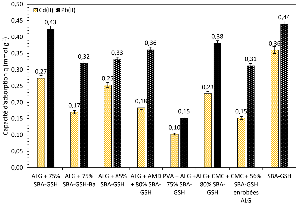
Figure 6.3 : Capacités d'adsorption de Cd(II) et Pb(II) par différentes billes contenant SBA-GSH et comparaison avec SBA-GSH en poudre ( C_0 = 4,5 \text{ mM} ; billes humides ( 10 \text{ g.L}^{-1} équivalent billes sèches) ; étude mono-élémentaire ; milieu \text{NaNO}_3 0,1 \text{ M} ; agitation magnétique 500 \text{ rpm} ; 25 \pm 1^\circ\text{C} ; 120 minutes de contact ; \text{pH} = 4 (Pb) ou 6,7 (Cd))
