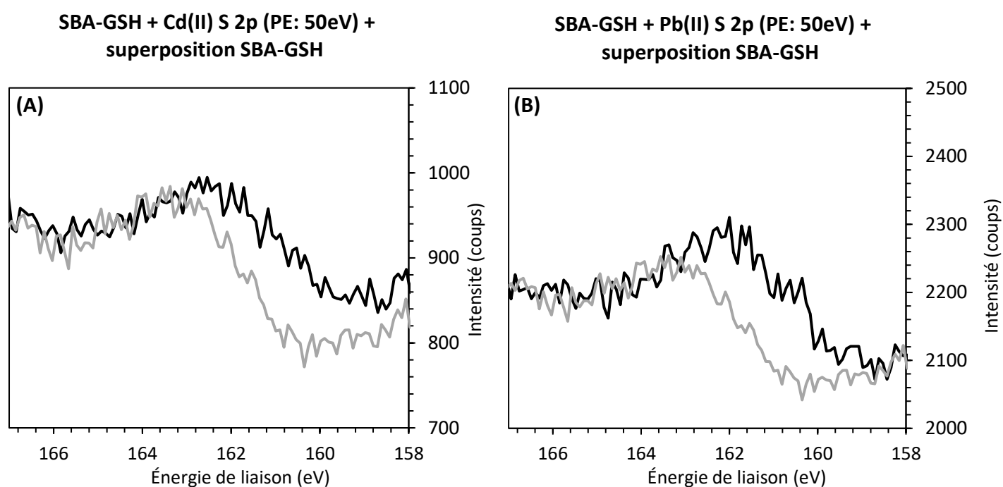
Figure 4.33 : Superposition des spectres XPS S 2p du matériau SBA-GSH avant adsorption (ligne claire) et après adsorption (ligne foncée) de Cd(II) (A) ou Pb(II) (B)
