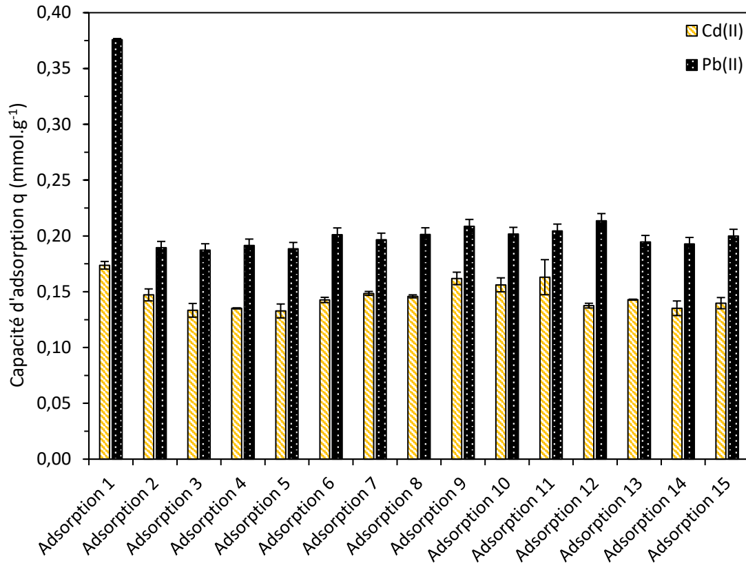
Figure 6.8 : Cycles adsorption/désorption de Cd(II) et Pb(II) sur les billes ALG + 75% SBA-GSH ( C_0 = 4,5 \text{ mM} ; billes humides ( 10 \text{ g.L}^{-1} équivalent billes sèches) ; matériau (masse sèche) ; étude mono-élémentaire ; agitation magnétique 500 rpm ; 25 \pm 1^\circ\text{C} ; 120 minutes de contact ; pH = 4 (Pb) ou 6,7 (Cd) ; désorption avec 0,01 \text{ M HNO}_3 + 0,1 \text{ M Ca(NO}_3)_2 )
