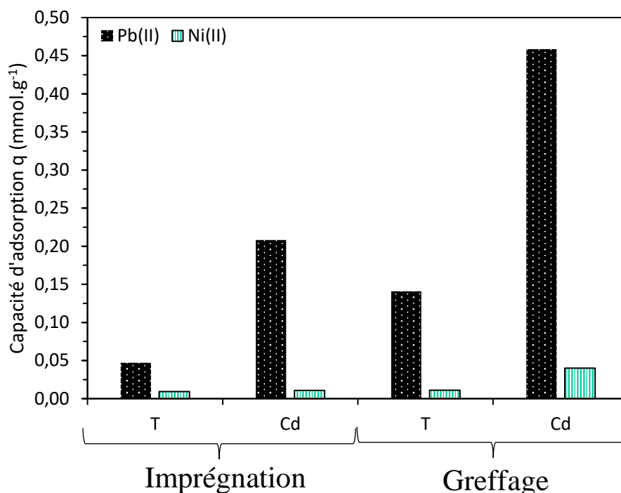
Figure 7.8 : Comparaison des matériaux SBA-LU-i et SBA-LU-g sur l'adsorption d'une solution bi-élémentaire PbNi ( C_0 = 4,5 mM par élément ; 10 g.L -1 de SBA-LU ; étude bi-élémentaire ; milieu NaNO 3 0,1 M ; agitation magnétique 500 rpm ; 25 \pm 1 °C ; 120 minutes de contact ; pH = 4,3 )
