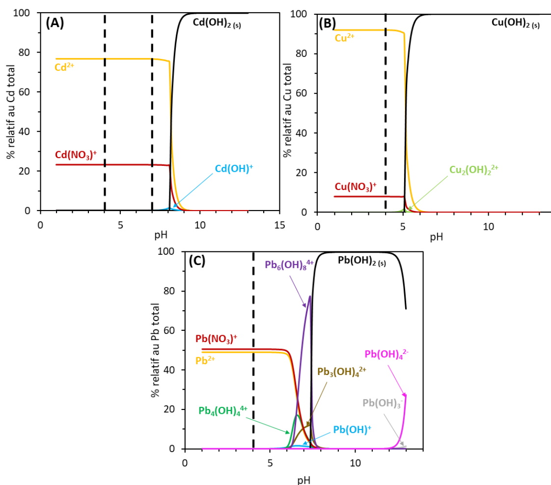
Figure 5.1 : Diagrammes de spéciation de Cd(II) (A), Cu(II) (B) et Pb(II) (C) ( [\text{M}(\text{II})] = 20 \text{ mM} ; [\text{NO}_3^-] = [\text{Na}^+] = 0,1 \text{ M} ; [\text{carbonates totaux}] = 1 \times 10^{-5} \text{ M} ; composés représentant au minimum 1% du M(II) total). Les lignes discontinues sont des indicateurs visuels des pH d'étude
