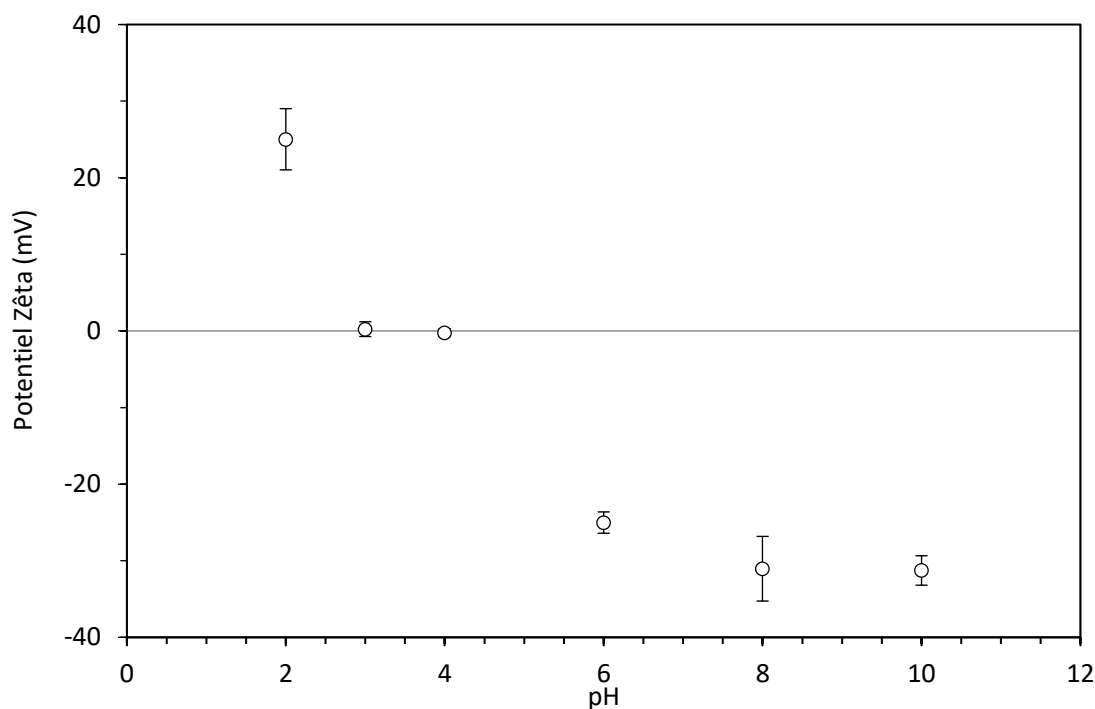
Figure 3.8 : Mesures du potentiel Zêta de SBA-GSH en fonction du pH (Milieu : \text{H}_2\text{O} ; 0,005% massiques de SBA-GSH ; 25 \pm 0,1^\circ\text{C} )
