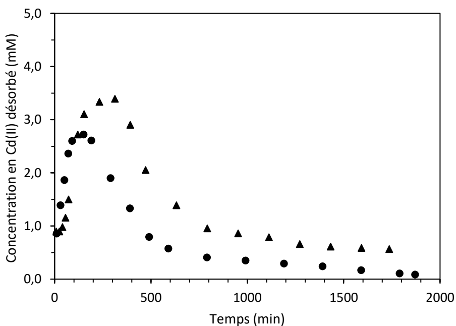
Figure 6.12 : Suivi de la concentration de Cd(II) désorbée par les billes ALG + 75% SBA-GSH dans la colonne aux débits 1 \text{ mL}\cdot\text{min}^{-1} (cercles) et 0,5 \text{ mL}\cdot\text{min}^{-1} (triangles) ( \text{HNO}_3 0,01 M + 0,1 M \text{Ca}(\text{NO}_3)_2 ; billes humides : 3,38 g de billes humides équivalent billes sèches ; étude mono-élémentaire ; 25 \pm 1^\circ\text{C} ; hauteur de lit 7,3 cm ; pH = 2)
