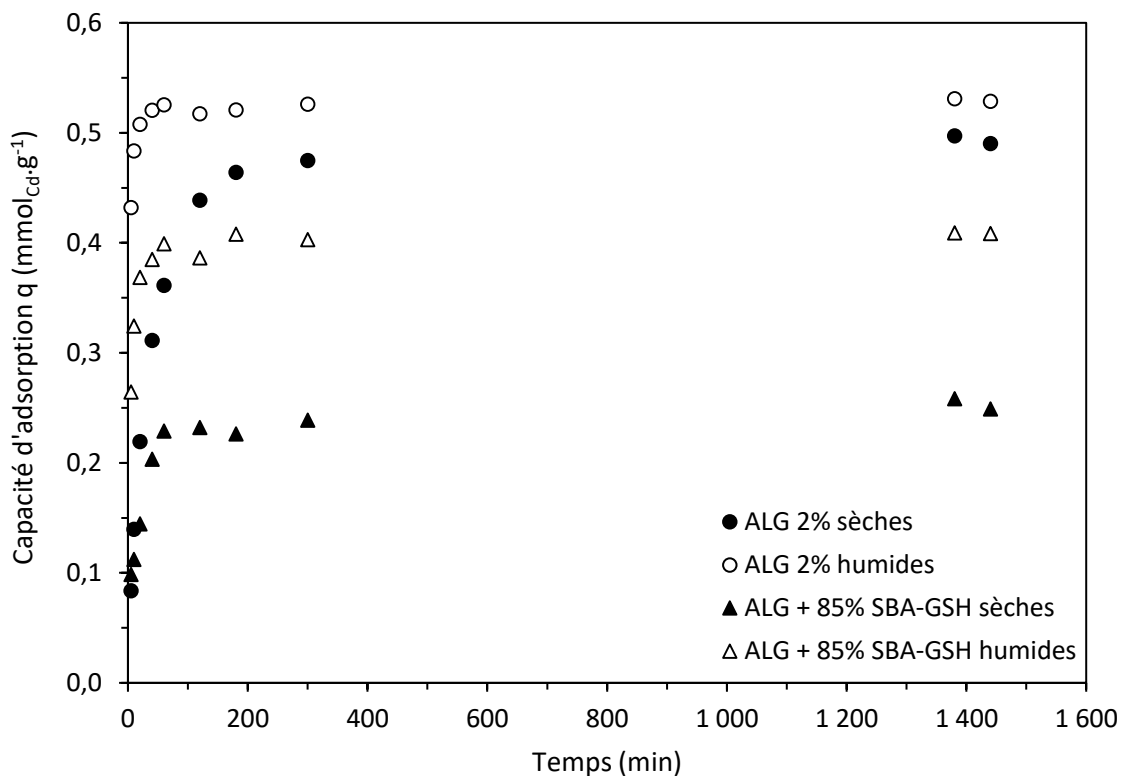
Figure 6.1 : Cinétiques d'adsorption de Cd(II) par des billes ALG 2% et ALG + 85% SBA-GSH humides et sèches ( C_0 = 8,0 \pm 0,5 \text{ mM}_{\text{Cd}} ; billes sèches ( 10 \text{ g.L}^{-1} ) ou billes humides ( 10 \text{ g.L}^{-1} équivalent billes sèches) ; étude mono-élémentaire ; milieu \text{NaNO}_3 0,1 \text{ M} ; agitation magnétique 500 \text{ rpm} ; 25 \pm 1^\circ\text{C} ; \text{pH} = 6,7 ). Erreur expérimentale : \leq 5\%
