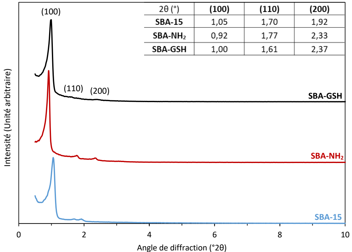
Figure 3.4 : Diffractogramme de rayons X aux bas angles des matériaux SBA-15, SBA-NH 2 et SBA-GSH
