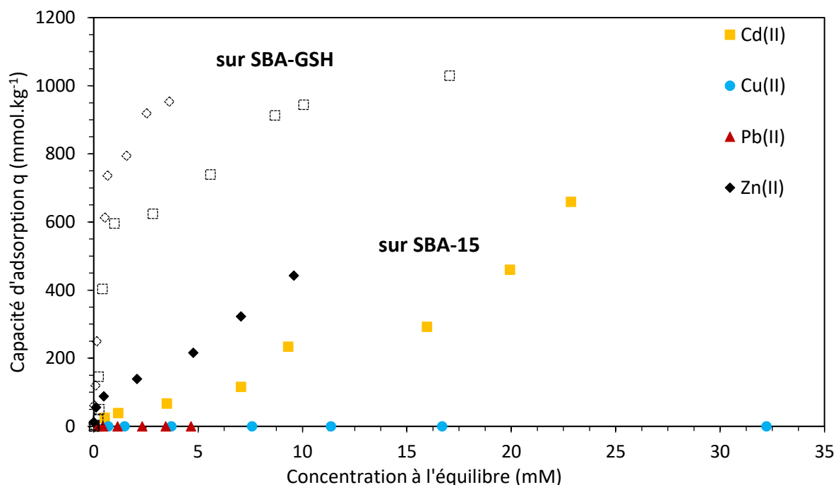
Figure 4.14 : Isothermes d'adsorption de Cd(II), Cu(II), Pb(II) et Zn(II) sur la silice SBA-15 non greffée et comparaison avec le matériau SBA-GSH ( C_0 = 0,08\text{-}20,4 \text{ mM}_{\text{Cd}} , 0,7\text{-}33,2 \text{ mM}_{\text{Cu}} , 0,2\text{-}4,6 \text{ mM}_{\text{Pb}} et 0,13\text{-}14,0 \text{ mM}_{\text{Zn}} ; 10 \text{ g.L}^{-1} de SBA-15 ; étude mono-élémentaire ; milieu \text{NaNO}_3 0,1 \text{ M} ; agitation magnétique 500 \text{ rpm} ; 25 \pm 1^\circ\text{C} ; 120 minutes de contact ; pH = 4 pour Cu(II) et Pb(II) et pH = 6,7 pour Cd(II) et Zn(II)). Les symboles ouverts représentent les isothermes (expérimentales) d'adsorption de Cd(II) (carrés) ou Zn(II) (losanges) sur SBA-GSH dans les mêmes conditions. Erreur expérimentale : \leq 2\% pour Cu(II) et Pb(II) et \leq 5\% pour Cd(II) et Zn(II)
