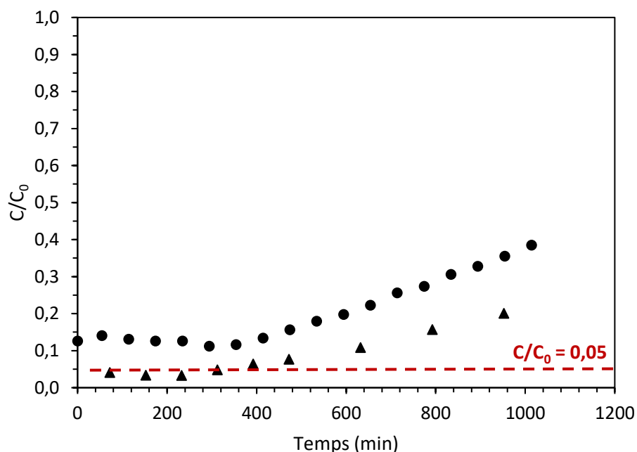
Figure 6.11 : Suivi du rapport C/C_0 représentant la proportion de Cd(II) adsorbé par les billes ALG + 75% SBA-GSH dans la colonne aux débits 1 \text{ mL}\cdot\text{min}^{-1} (cercles) et 0,5 \text{ mL}\cdot\text{min}^{-1} (triangles) ( C_0 = 1 \text{ mM} ; billes humides : 3,38 g de billes humides équivalent billes sèches ; étude mono-élémentaire ; 25 \pm 1^\circ\text{C} ; hauteur de lit 7,3 cm ; pH = 6,6)
