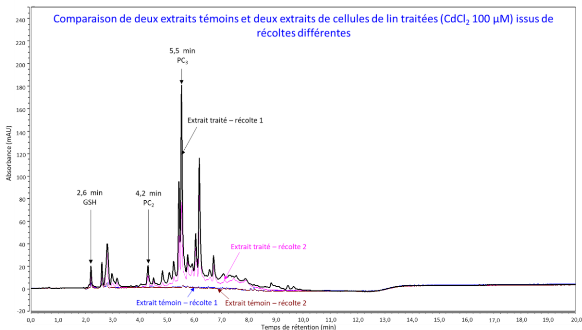
Figure 7.5 : Comparaison par analyse UHPLC-UV de la composition des extraits de cellules de lin témoin et traitées avec CdCl 2 100 μM sur deux cultures différentes espacées de 14 jours
