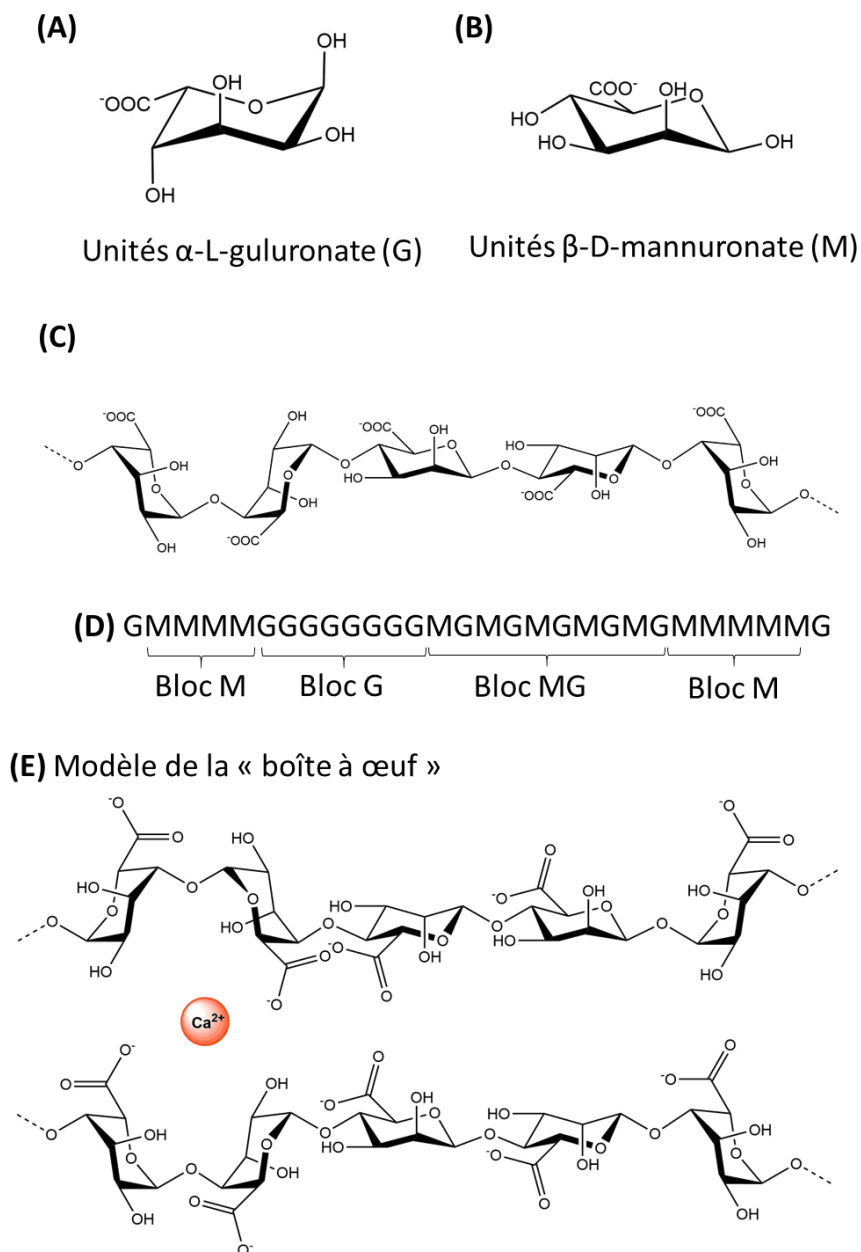
Figure 1.9 : Structure des monomères G (A) et M (B) de l'alginate, de la conformation macromoléculaire de l'alginate (C), schéma des différents blocs (D) et modèle de la « boîte à œuf »
