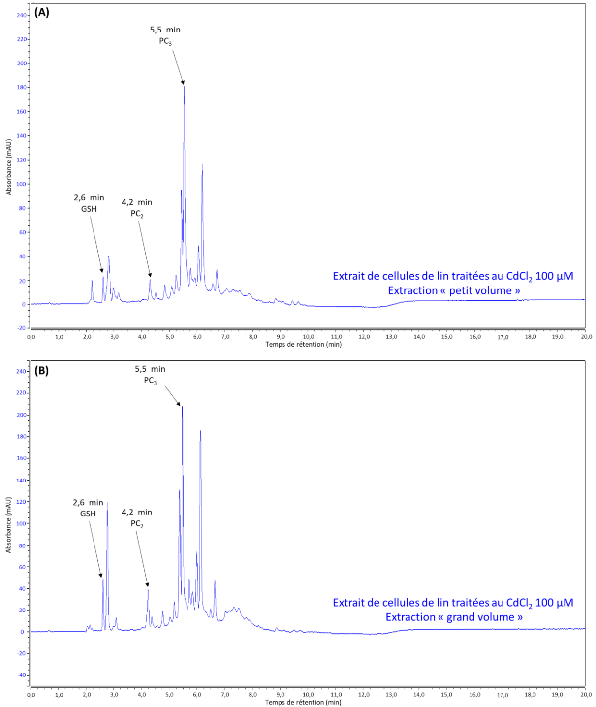
Figure 7.1 : Comparaison de la composition des extraits de cellules de lin traitées par du \text{CdCl}_2 100 \mu\text{M} pendant 14 jours, issus des protocoles d'extraction « petit volume » (A) et « grand volume » (B) par analyse UHPLC-UV
