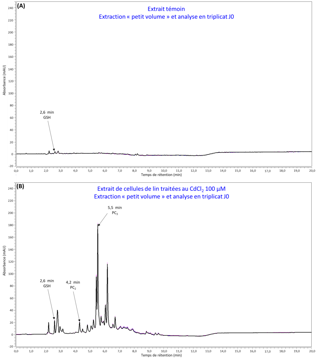
Figure 7.4 : Comparaison par analyse UHPLC-UV en triplicat de la composition des extraits de cellules de lin témoin (A) ou traitées au CdCl 2 100 μM pendant 14 jours (B)
