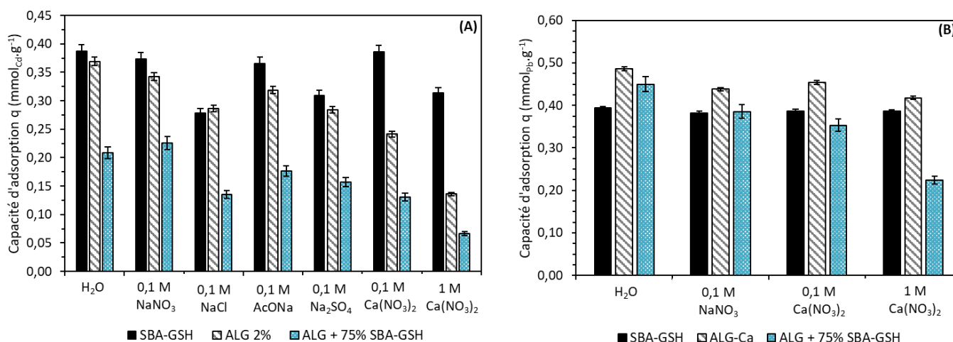
Figure 6.6 : Suivi de la capacité d'adsorption de Cd(II) (A) et Pb(II) (B) en fonction de la présence de différents sels ( C_0 = 4,5 \text{ mM} ; billes humides ( 10 \text{ g.L}^{-1} équivalent billes sèches) ; étude mono-élémentaire ; agitation magnétique 500 rpm ; 25 \pm 1^\circ \text{C} ; 120 minutes de contact ; pH = 4 (Pb) ou 6,7 (Cd))
