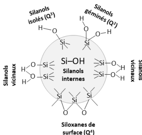
Figure 1.5 : Sites à la surface d'une silice mésoporeuse
