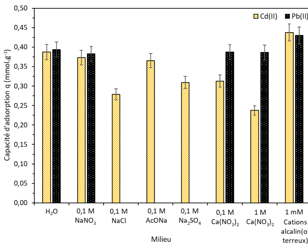
Figure 4.6 : Suivi de la capacité d'adsorption de Cd(II) et Pb(II) en fonction de la présence de différents sels ( C_0 = 4,5 \text{ mM} ; 10 \text{ g} \cdot \text{L}^{-1} de SBA-GSH ; étude mono-élémentaire ; agitation magnétique 500 rpm ; 25 \pm 1^\circ\text{C} ; 120 minutes de contact ; pH = 4 (Pb) ou 6,7 (Cd))
