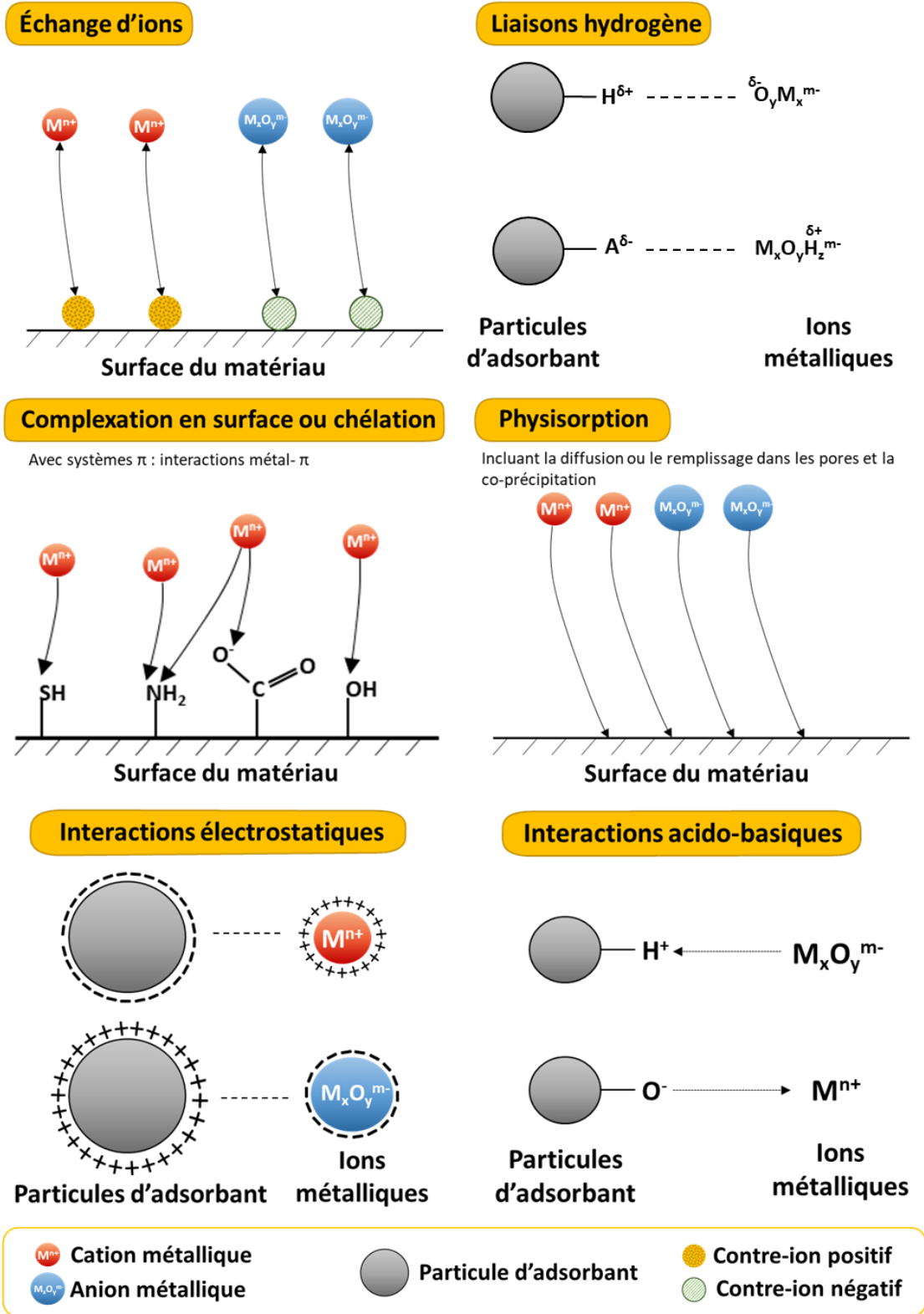
Figure 1.8 : Interactions possibles entre des composés métalliques ioniques et un matériau adsorbant. Les écritures M^{n+} et M_xO_y^{m-} sont des simplifications et les interactions sont considérées pour tout complexe ionique d'ion métallique
