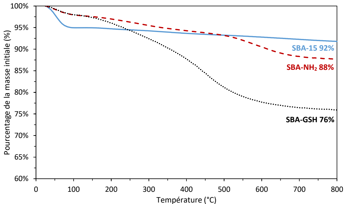
Figure 3.9 : Analyse thermogravimétrique des matériaux SBA-15, SBA-NH 2 et SBA-GSH
