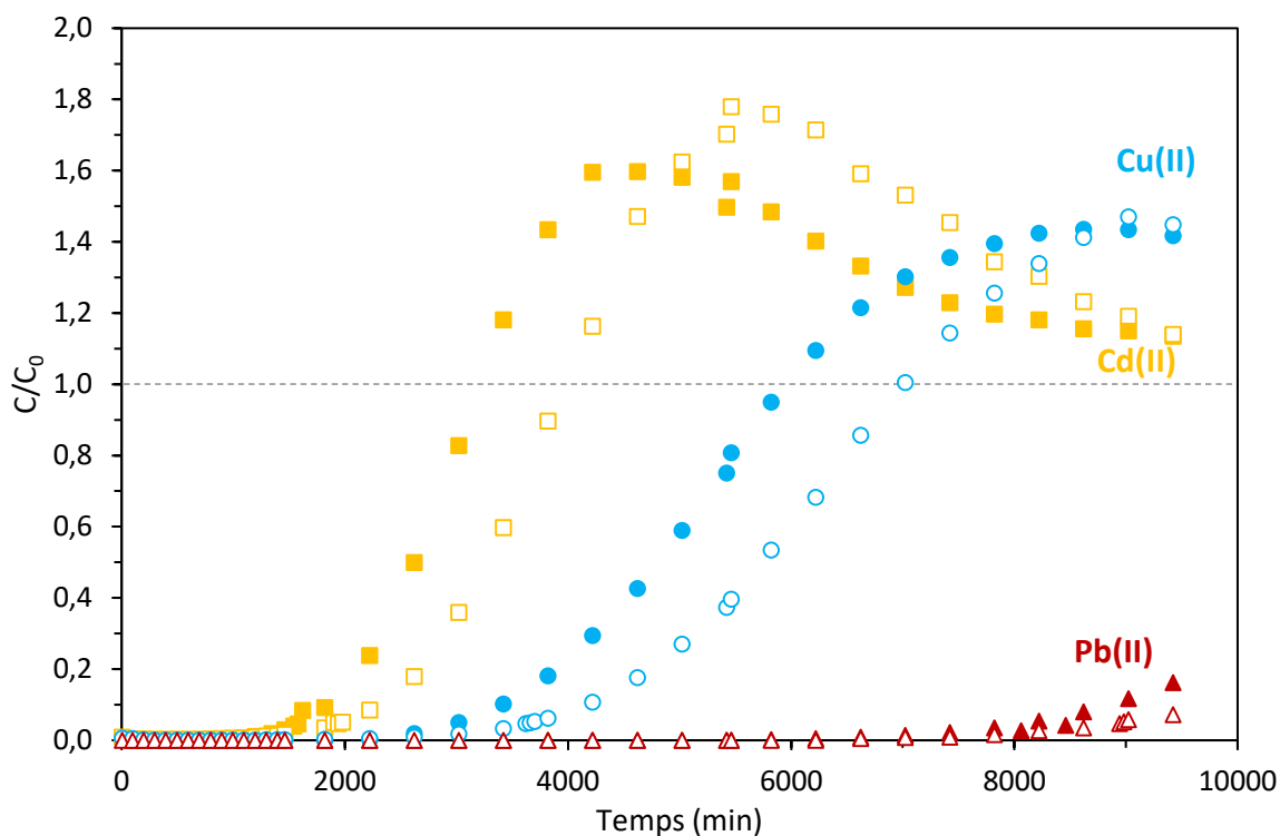
Figure 6.17 : Courbes de percée de l'adsorption du mélange CdCuPb sur les billes ALG + 75% SBA-GSH-Ba ( C_0 = 1 mM totale ; 4,46 g de billes humides équivalent billes sèches ; étude tri-élémentaire ; 25 \pm 1^\circ\text{C} ; hauteur de lit 7,2 cm ; pH = 4,7). Les symboles vides représentent les données des billes gélifiées dans Ca 2+ et les symboles pleins celles des billes gélifiées dans Ba 2+
