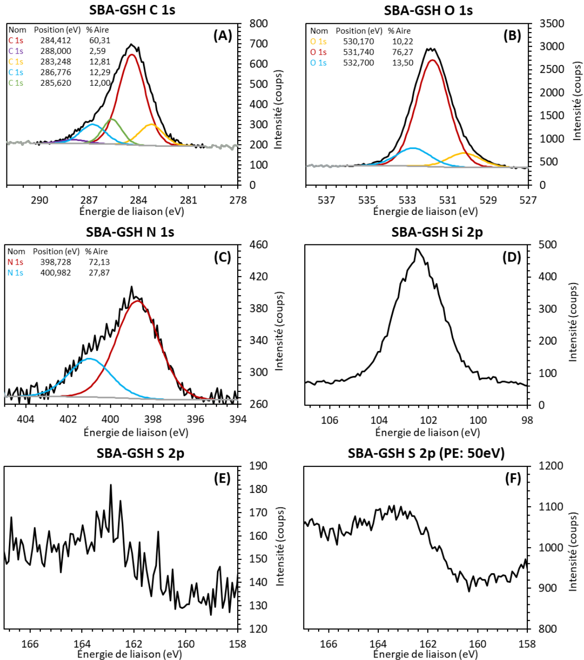
Figure 3.12 : Spectres XPS du matériau SBA-GSH (A) C 1s, (B) O 1s, (C) N 1s, (D) Si 2p, (E) S 2p et (F) S 2p (PE : 50 eV)
