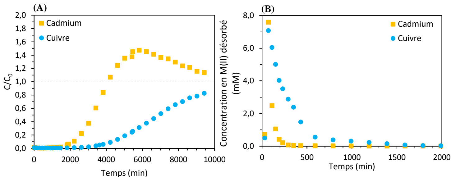
Figure 6.15 : Courbes de percée de l'adsorption (A) et de la désorption (B) du mélange CdCu sur les billes ALG + 75% SBA-GSH ( C_0 = 1 \text{ mM} totale (Adsorption) ou éluant \text{HNO}_3 \text{ } 0,01 \text{ M} + 0,1 \text{ M Ca(NO}_3)_2 (Désorption) ; 4,54 g de billes humides équivalent billes sèches ; étude bi-élémentaire ; 25 \pm 1^\circ\text{C} ; hauteur de lit 7,8 cm ; \text{pH} = 4,7 )
