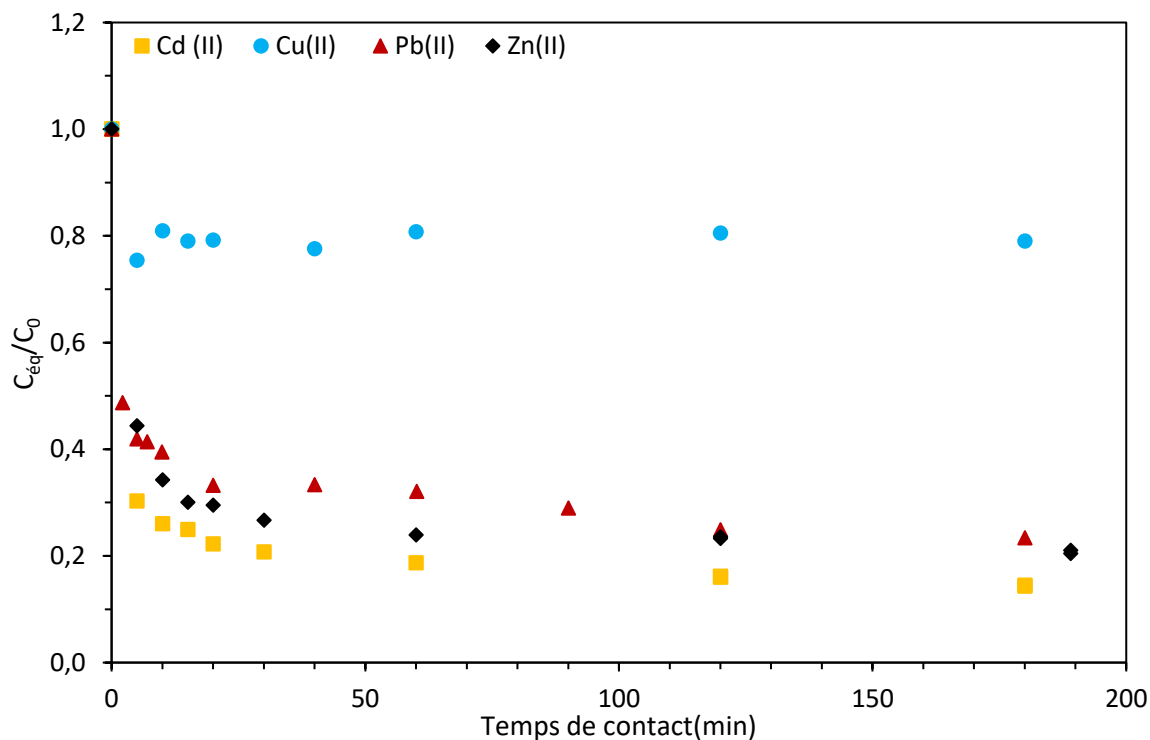
Figure 4.7 : Étude cinétique de l'adsorption de Cd(II), Cu(II), Pb(II) et Zn(II) par SBA-GSH : suivi temporel du rapport C_{éq}/C_0 ( C_0 = 8 \pm 0,5 mM pour chacun des ions métalliques ; 10 \text{ g.L}^{-1} de SBA-GSH ; étude mono-élémentaire ; milieu \text{NaNO}_3 0,1 \text{ M} ; agitation magnétique 500 \text{ rpm} ; 25 \pm 1^\circ\text{C} ; \text{pH} = 4 ou 6,7 pour Cu(II)/Pb(II) ou Cd(II)/Zn(II) respectivement). Erreur expérimentale sur C_{éq}/C_0 : \pm 0,05 pour Pb(II) et Cd(II) ; \pm 0,02 pour Zn(II) et \pm 0,01 pour Cu(II)
