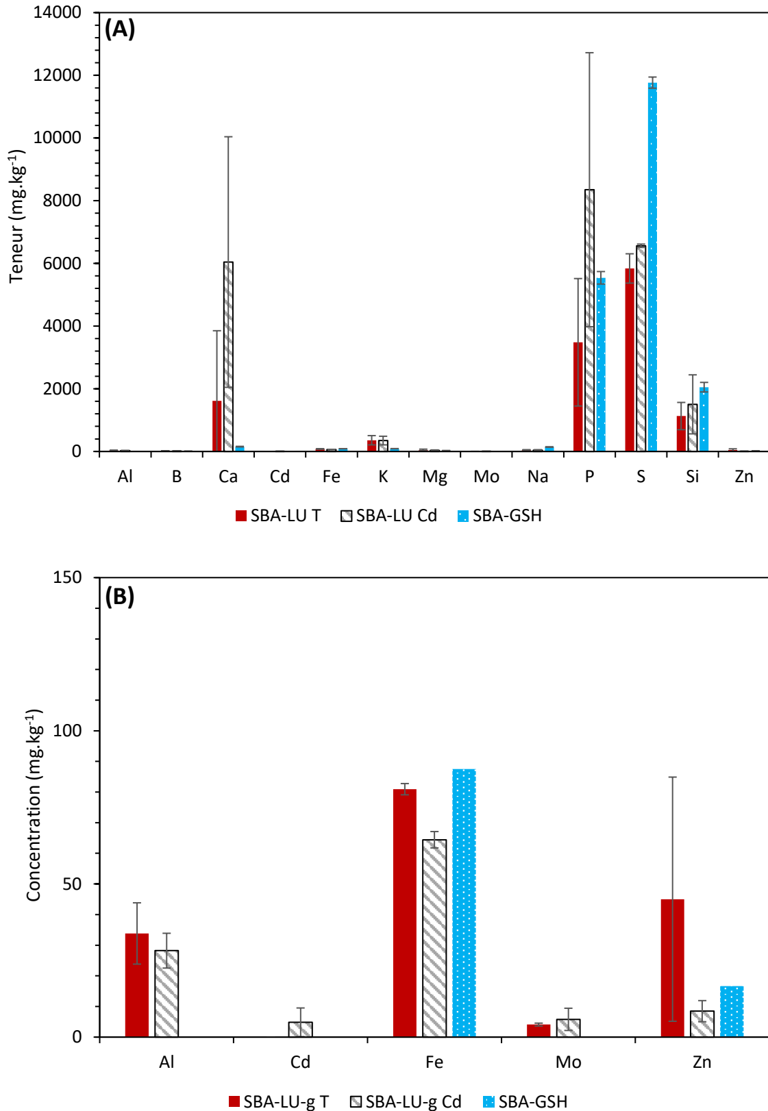
Figure 7.11 : Analyse par ICP-AES des éléments contenus dans les matériaux SBA-LU-g T, SBA-LU-g Cd et comparaison avec SBA-GSH : représentation de l'ensemble des éléments détectés (A) et éléments métalliques de transition et aluminium (B)
