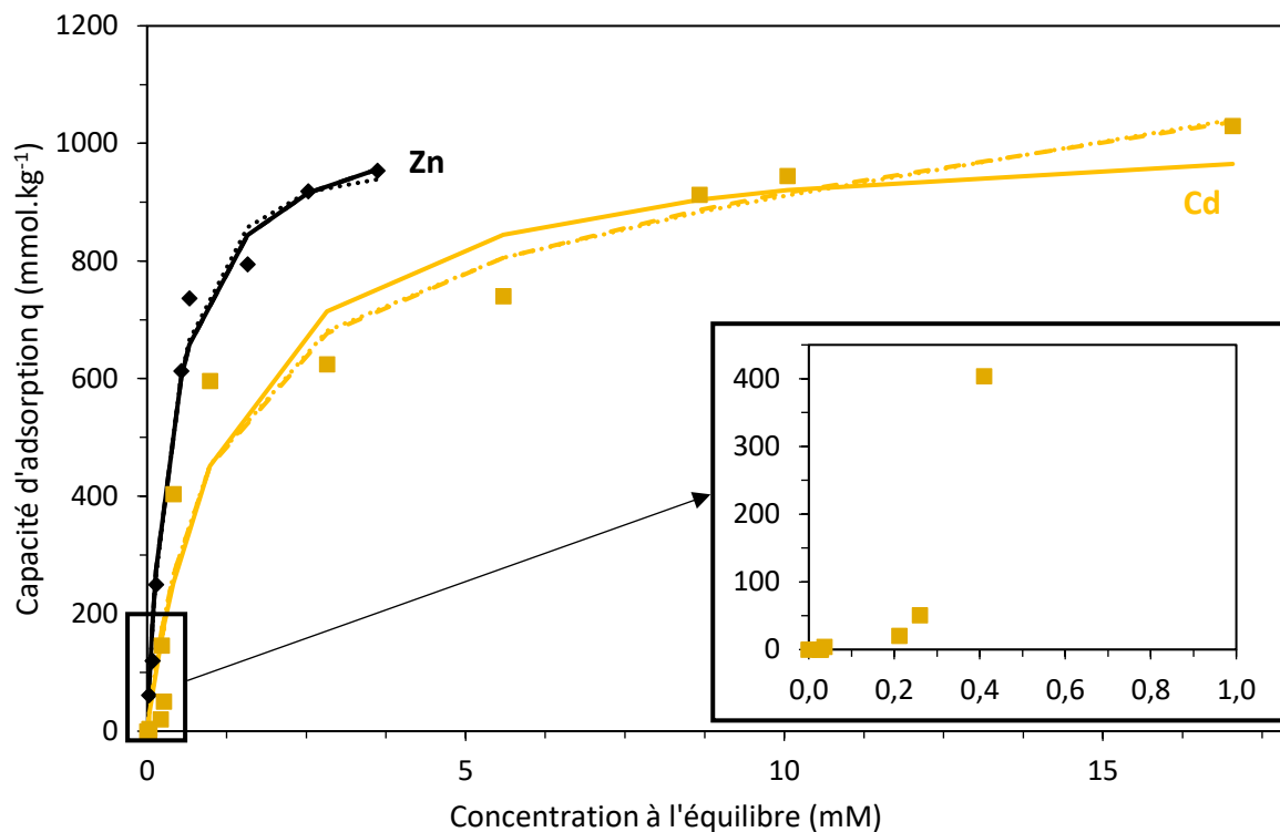
Figure 4.12 : Isothermes d'adsorption de Cd(II) et Zn(II) sur le matériau SBA-GSH ( C_0 = 0,0004-26,7 \text{ mM}_{\text{Cd}} et 0,66-26,5 \text{ mM}_{\text{Zn}} ; 10 \text{ g.L}^{-1} de SBA-GSH ; étude mono-élémentaire ; milieu \text{NaNO}_3 0,1 \text{ M} ; agitation magnétique 500 \text{ rpm} ; 25 \pm 1^\circ\text{C} ; 120 minutes de contact ; \text{pH} = 6,7 ) et agrandissement sur les points de faibles concentrations initiales en Cd(II) ( C_0 = 0,0004-2 \text{ mM} ). Les symboles représentent les valeurs expérimentales, la ligne continue le modèle de Langmuir, les tirets le modèle de Langmuir bi-site et les points le modèle BET. Erreur expérimentale : \leq 3\% pour Cd(II) et \leq 6\% pour Zn(II)
