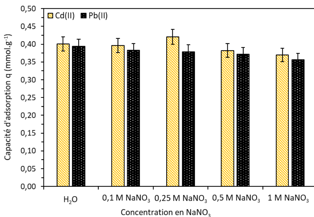
Figure 4.5 : Suivi de la capacité d'adsorption de Cd(II) et Pb(II) en fonction de la concentration en NaNO 3 ( C_0 = 4,5 \text{ mM} ; 10 \text{ g} \cdot \text{L}^{-1} de SBA-GSH ; étude mono-élémentaire ; agitation magnétique 500 rpm ; 25 \pm 1^\circ\text{C} ; 120 minutes de contact ; pH = 4 (Pb) ou 6,7 (Cd))
