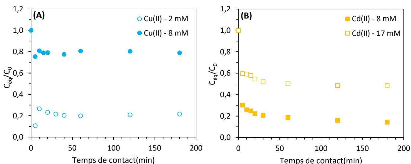
Figure 4.8 : Étude cinétique de l'adsorption de Cu(II) (A) et Cd(II) (B) à différentes concentrations par SBA-GSH : suivi temporel du rapport C_{éq}/C_0 (10 g.L -1 de SBA-GSH ; étude mono-élémentaire ; milieu NaNO 3 0,1 M ; agitation magnétique 500 rpm ; 25 ± 1°C ; pH = 4 (Cu) ou 6,6 (Cd)). Erreur expérimentale sur C_{éq}/C_0 : ± 0,01 pour Cu(II) et ± 0,04 pour Cd(II)
