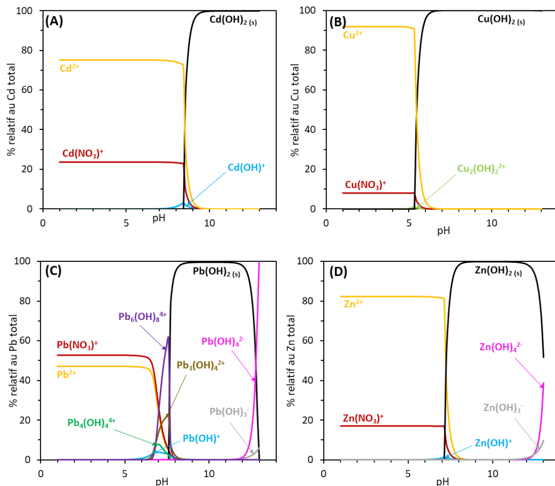
Figure 4.1 : Diagrammes de spéciations de Cd(II) (A), Cu(II) (B), Pb(II) (C) et Zn(II) (D) ( [\text{M}(\text{II})] = 4,5 \text{ mM} ; [\text{NO}_3^-] = 0,1 \text{ M} ; [\text{Na}^+] = 0,1 \text{ M} et [\text{carbonates totaux}] = 1 \times 10^{-5} \text{ M} ; composés représentant au minimum 1% du M(II) total)
