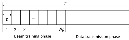
Figure 7: L'intervalle de temps d'une durée de T comprend : (i) une phase d'apprentissage du faisceau, qui consiste en N_b^2 mini-créneaux d'une durée de \tau ; (ii) une phase de transmission des données.
