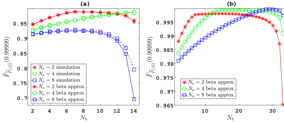
Figure 8: Proportion de dispositifs ayant une probabilité de couverture du débit conditionnel effective supérieure au seuil de fiabilité 99.999% en fonction du nombre de faisceaux pour T = 1 ms (a) et T = 5 ms (b).
