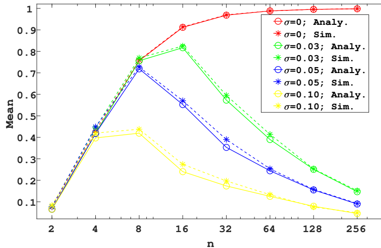
Figure 5: Moyenne de P_s(\eta) en fonction du nombre d'antennes n pour différents écarts d'erreur d'alignement \epsilon .
