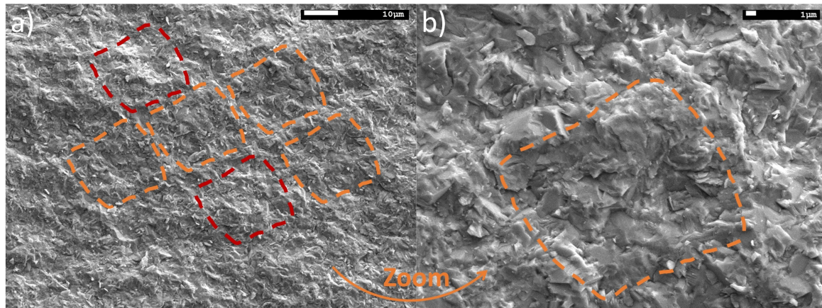
Figure IV-63 : Cliché réalisé au MEB de la surface de rupture de GC-1200 après un essai DCDC.
