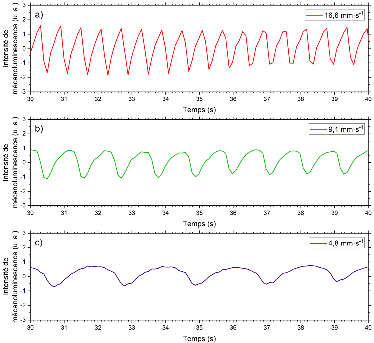
Figure IV-66 : Mécanoluminescence de GC-1200 lorsque l'échantillon est rayé avec une charge de 6,3 N, avec une vitesse de déplacement de l'indenteur de a) 16,6 mm·s -1 , b) 9,1 mm·s -1 , et c) 4,8 mm·s -1 .
