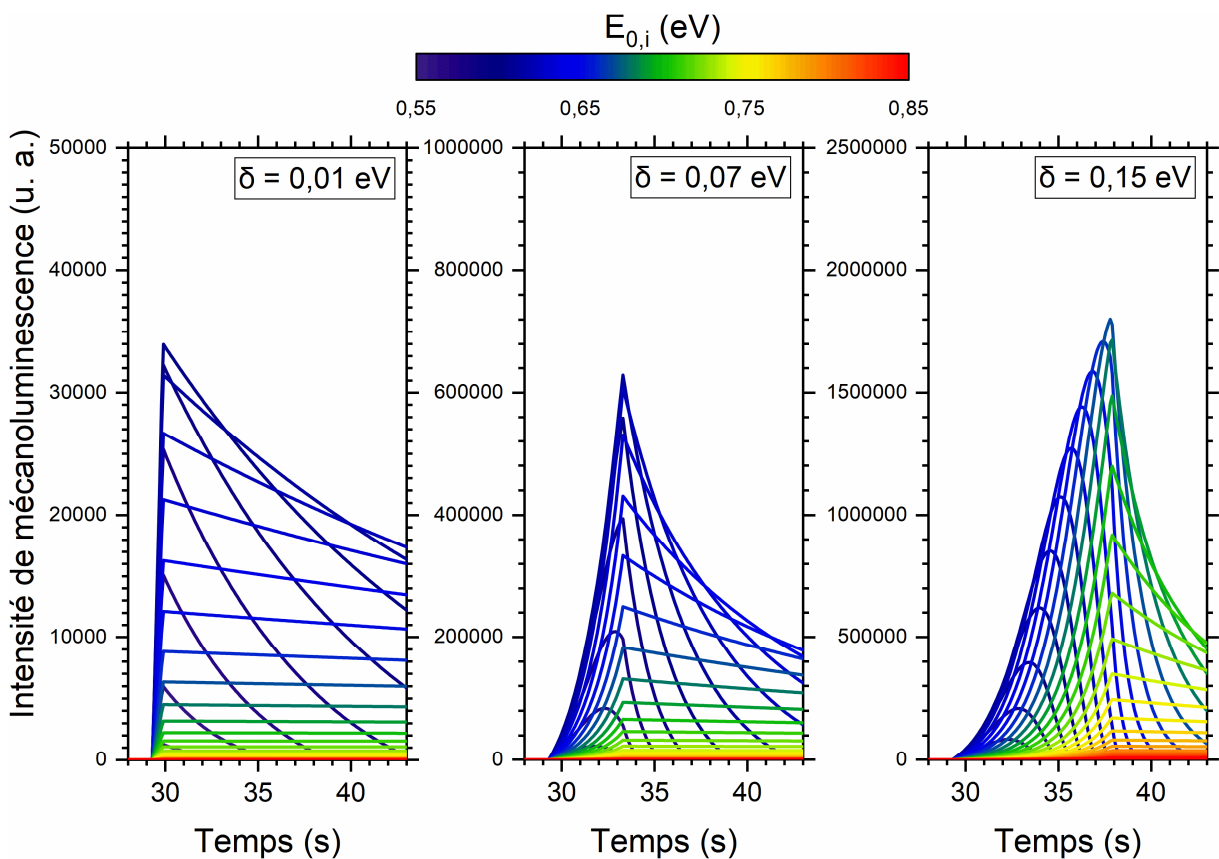
Figure IV-54 : Intensité de mécanoluminescence calculée pour chaque piège discret i avec \dot{\delta} = 0,0175 \text{ eV}\cdot\text{s}^{-1} , pour \delta = 0,01 \text{ eV} (gauche), \delta = 0,07 \text{ eV} (milieu) et \delta = 0,15 \text{ eV} (droite).
