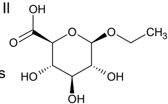
Figure 7: Molécule d'EtG
