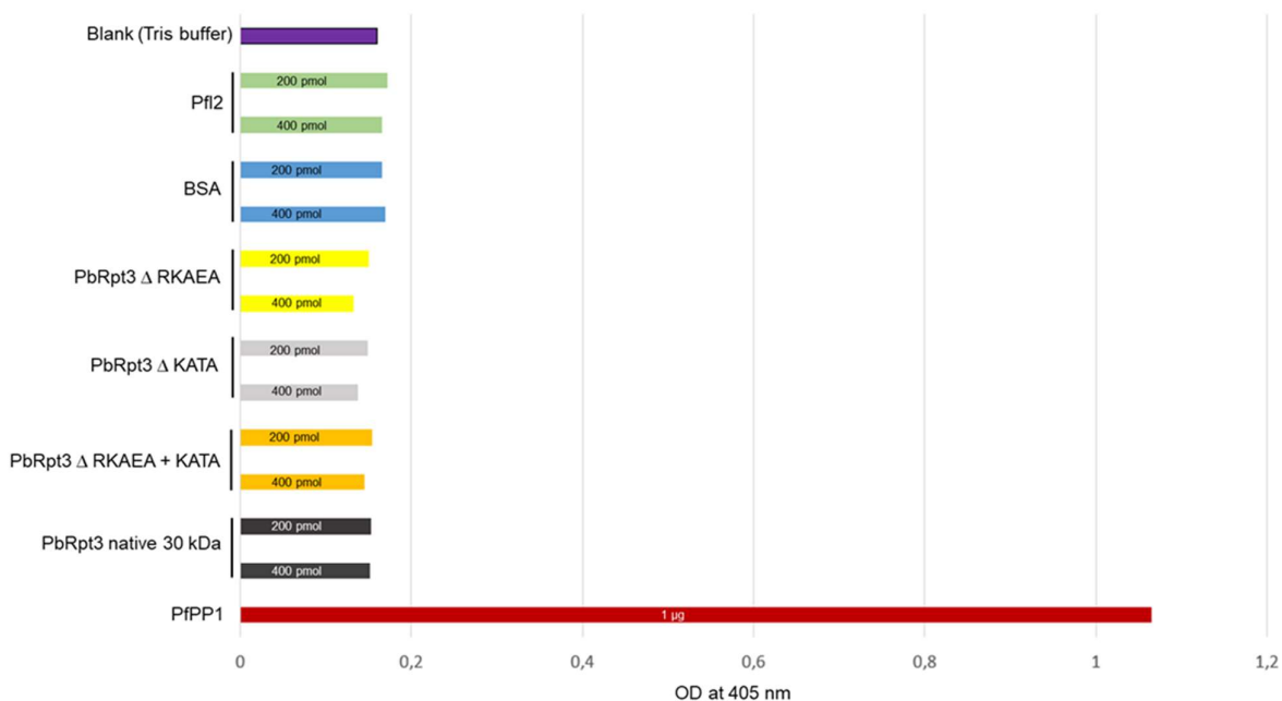
Figure 47. Etude de l'activité phosphatase de PRpt3-30 kDa, des différentes protéines mutées sur les motifs RVxF, ainsi que des protéines contrôle BSA, Pfi2 et PfPP1c grâce à un test pNPP. Différentes quantités de chaque protéine (200 ou 400 pmol), ou 1 μg de PfPP1c recombinante ont été incubées avec le substrat pNPP pendant 1 heure à 37°C. Les résultats sont présentés en valeurs de Densité Optique à 450 nm.
