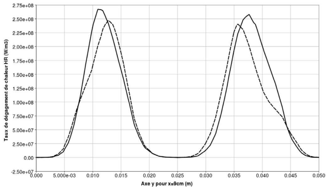
FIG. 9.14 – Profils de taux de dégagement de chaleur le long de l'axe y = 2 cm, z = 0 pour les simulations avec (trait pointillé) et sans rayonnement (trait continu).
