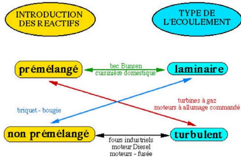
FIG. 1.2 – Systèmes pratiques classés selon le type d'injection (prémélangée ou non) et la nature laminaire ou turbulente de l'écoulement, d'après [8].
