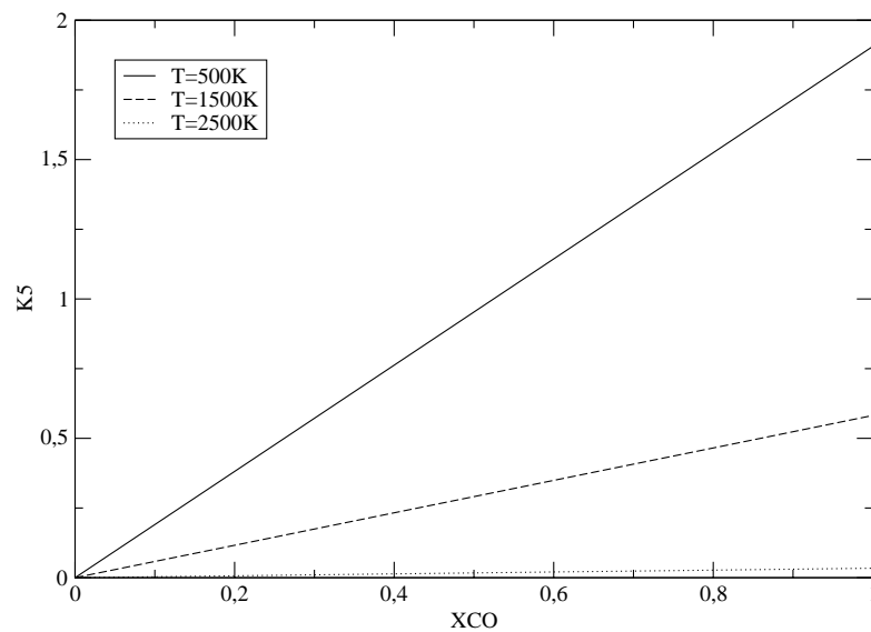
FIG. A.4 – Variation de \kappa_5 avec la fraction molaire de \text{CO} pour T = 500, 1500 et 2500\text{K} .
