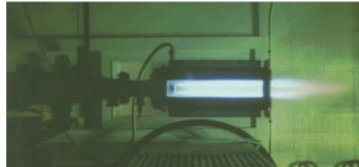
FIG. 8.2 – Photo du dispositif expérimental de l'EM 2 C (allumé) [125, 126, 127, 123].
