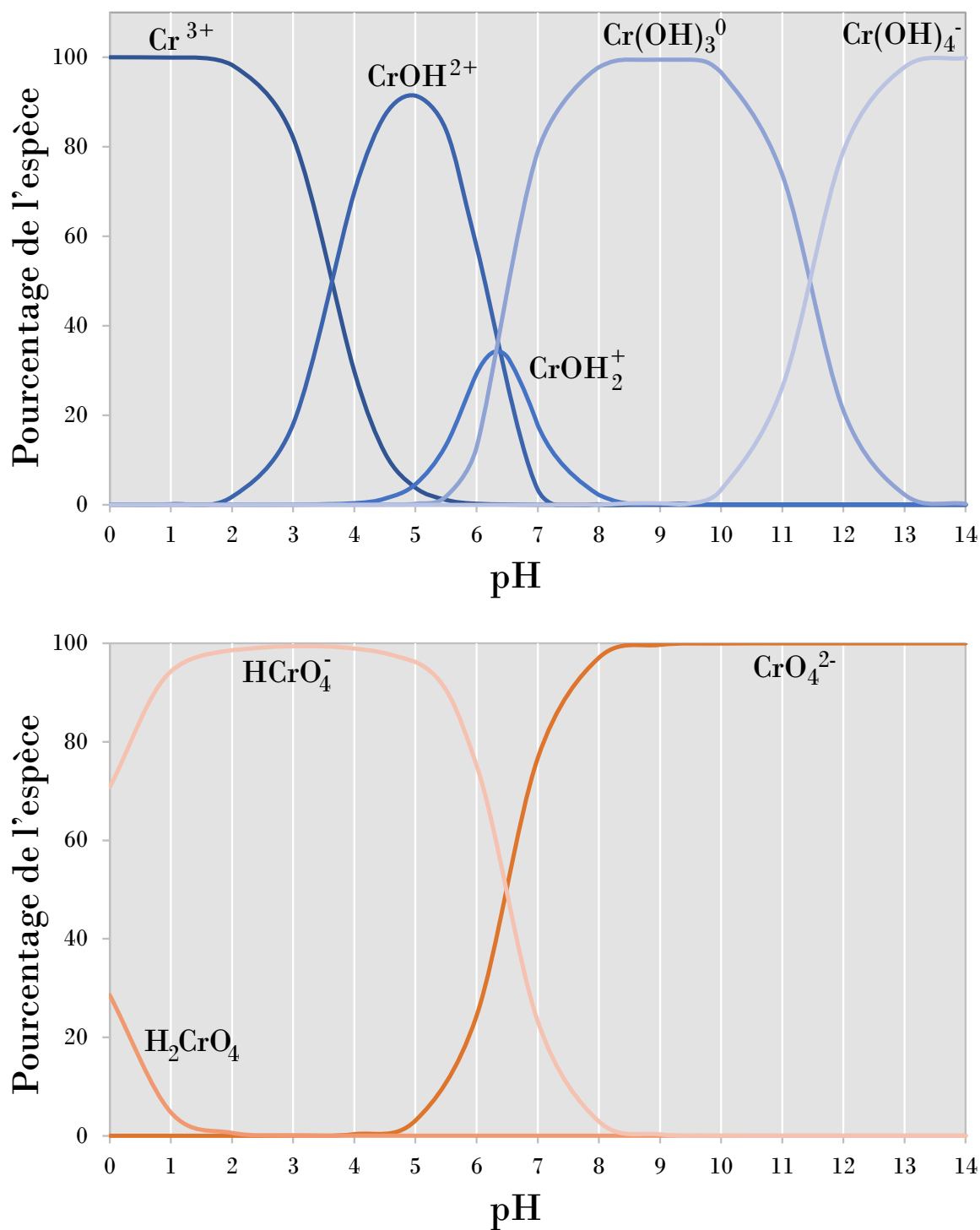
Figure 4.6 | Distribution des espèces de Cr(III) et Cr(VI) selon le pH, pour [\text{Cr}] = 200 \mu\text{mol/L} . Réalisé avec Visual MINTEQ 3.1.
