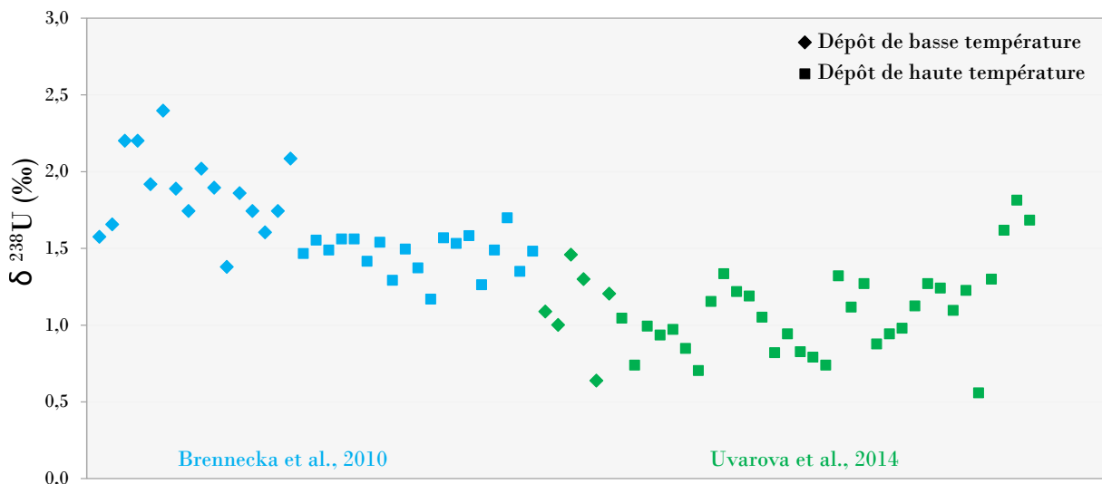
Figure 6.1 | Valeurs de \delta^{238}U (VS CRM-129 A) selon le type de dépôt, publiées par Brennecka et al. (2010) et Uvarova et al. (2014). On observe que les valeurs mesurées par Uvarova et al. (2014) ne présentent pas de différence significative entre dépôts de haute et de basse température, ne permettant pas de discriminer le type de dépôt selon ce paramètre.
