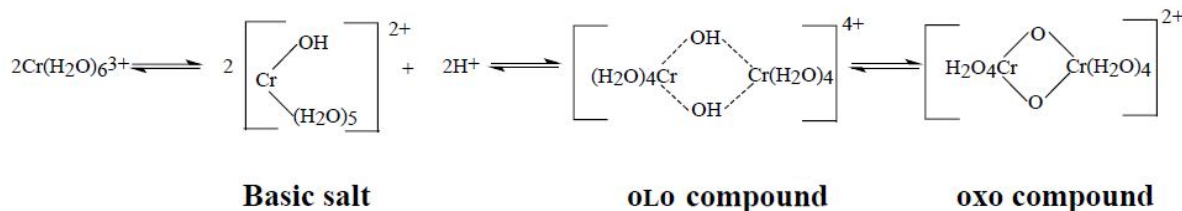
Figure 5.3 | Formation d'oxo-composés à partir de sels de chrome. D'après [Mann and McMillan (2017)].
