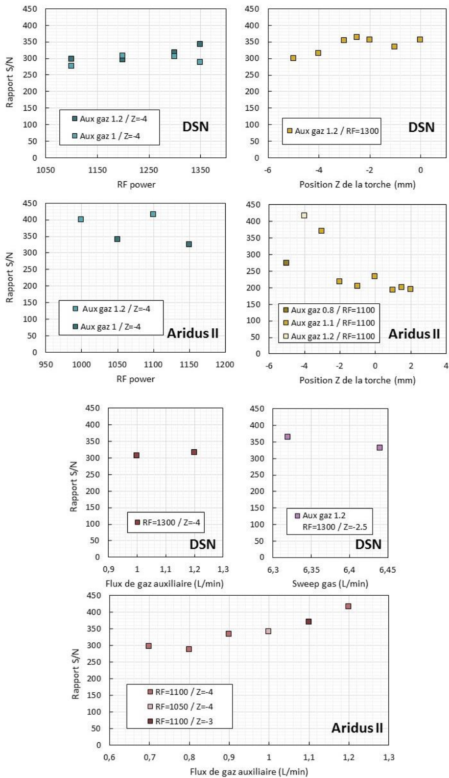
Figure 10 : Valeur du rapport signal sur bruit (S/N) en fonction de la valeur du RF power, de la position en Z de la torche et de différents flux de gaz avec le DSN et l'Aradius II.
