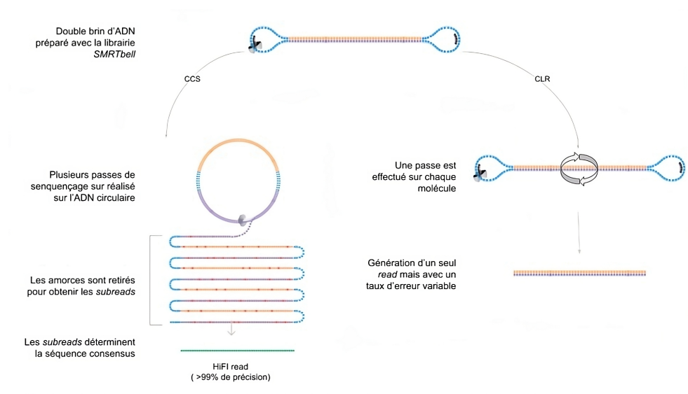
FIGURE 1.21 – Présentation des différents modes du séquençage PacBio Deux modes principaux : Circular Consensus Sequencing (CCS) et Continuous Long Read (CLR).
