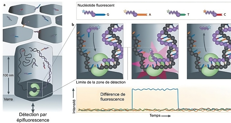
FIGURE 1.20 – Séquençage PacBio Adapté selon RNA-Seq blog
