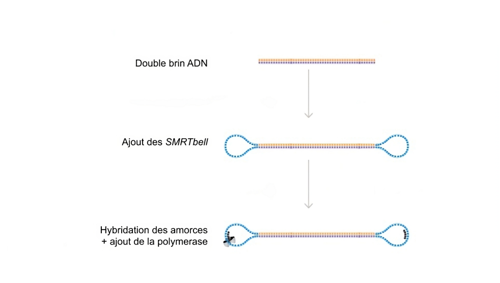
FIGURE 1.19 – Présentation de la librairie SMRT bell
