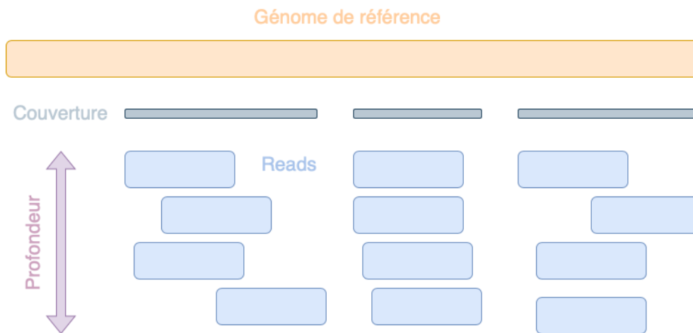
FIGURE 1.23 – Représentation d’un alignement de reads Lorsque des reads sont alignés à un génome de référence, on les nomme reads alignés.
