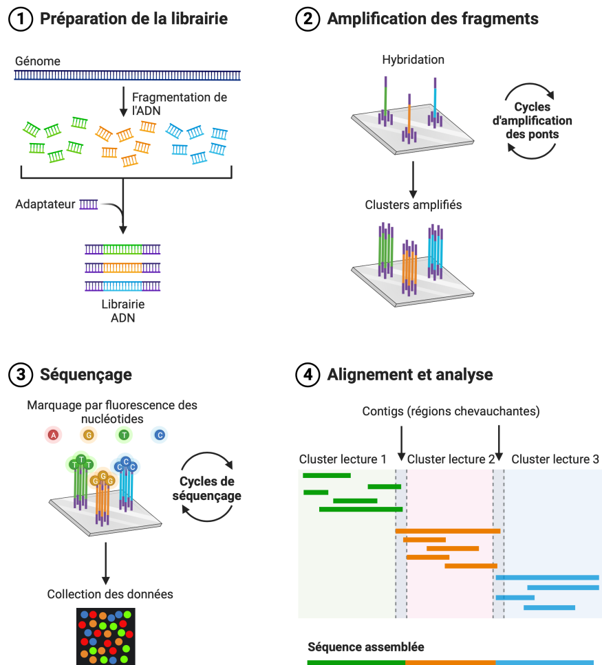
FIGURE 1.17 – Séquençage Illumina Séquençage Illumina d’une librairie ADN. Adapté de Next Generation Sequencing, BioRender
