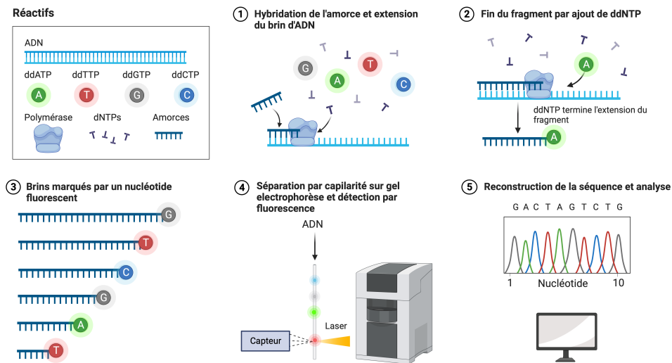
FIGURE 1.14 – Le Séquençage Sanger
