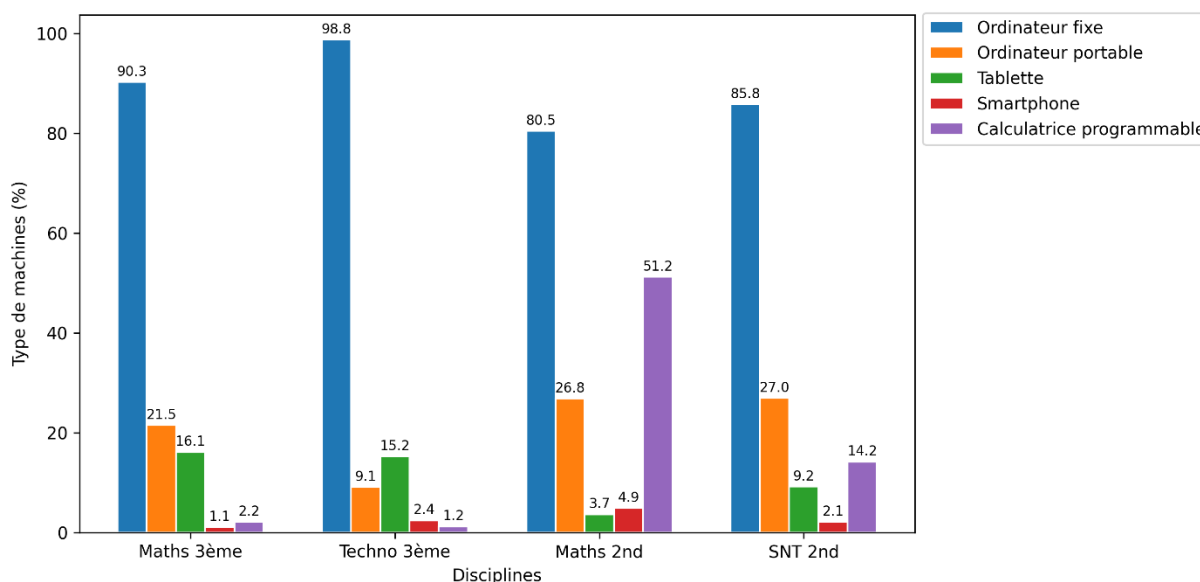
Figure 4-25 – Types de machines utilisées par les élèves pour programmer en proportion et par disciplines / QF3 : Quel type de machine vos élèves utilisent-ils pour développer leurs programmes informatiques ?
