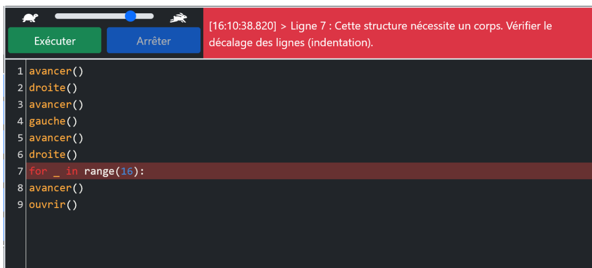
Figure 5-26 – Détail de l'interface utilisateur de Pyrates lors de la survenue d'une erreur syntaxique : message d'erreur et mise en valeur de la ligne erronée
