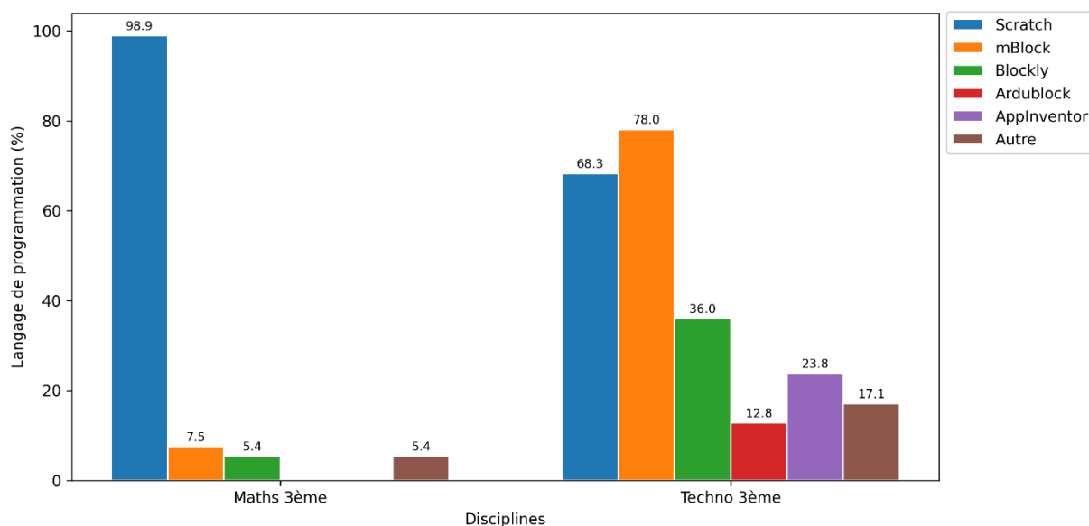
Figure 4-26 – Langages de programmation utilisés par les élèves en proportion par discipline du collège / QF8 : Quel(s) langage (s) de programmation graphique vos élèves utilisent-ils ?
