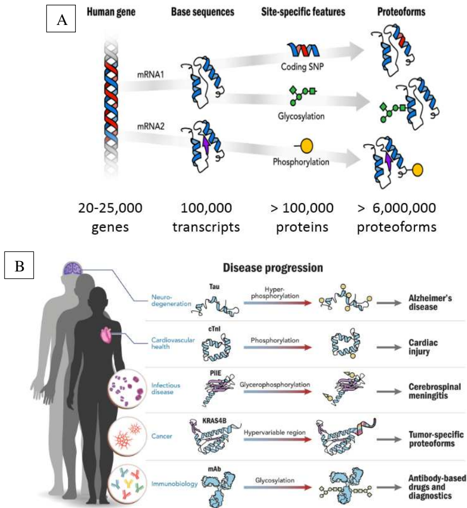
Figure 18 : A : Différentes protéoforment issues d'un même gène 178 . B : exemples de rôle de protéoforment dans la progression de maladies chez l'homme 178 .
