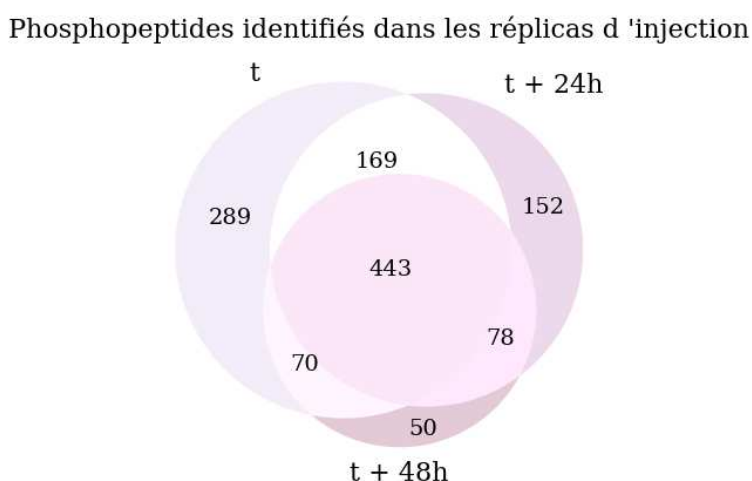
Figure 53 : Recouvrement des phosphopeptides entre les 3 répliques d'injection.
