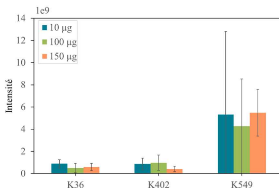
Figure 109 : Intensité moyenne dans les échantillons enrichis avec les dépôts de 10 \mu\text{g} (N=2, les barres d'erreurs ont été illustrées grâce à un écart-type standard calculé sur Excel), 100 \mu\text{g} (N=3) et 150 \mu\text{g} (N=3) sur les lysines 36, 402 et 549.
