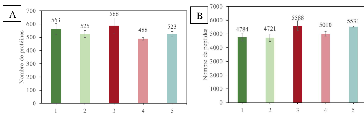
Figure 49 : Nombre moyen de protéines (A) et de peptides (B) identifiés par analyse LC-MS/MS à partir des différentes extractions : 1 = Urée, 2 = Urée avec précipitation, 3 = Urée/thio-urée, 4 = Urée/thio-urée avec précipitation et 5 = Laemmli-like.
