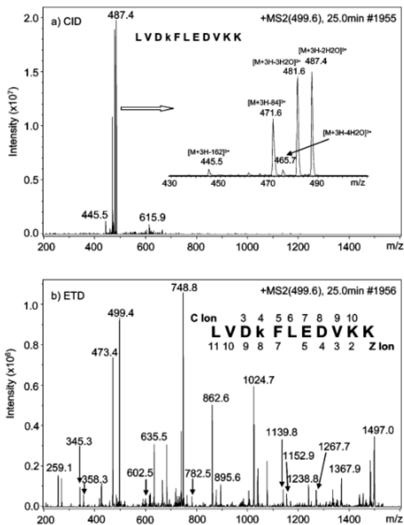
Figure 35 : Spectres de fragmentation du peptide LVK FLEDVKK après fragmentation par CID ou par ETD 276 .
