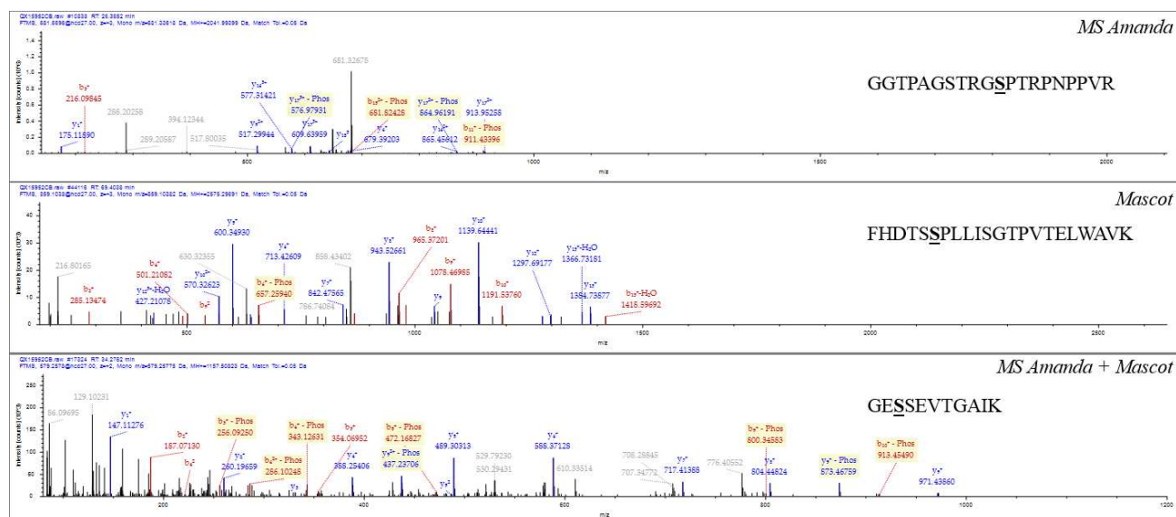
Figure 61 : Spectres de peptides phosphorylés identifiés par MS Amanda seul, Mascot seul et identifiés par les deux logiciels.
