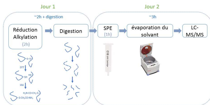
Figure 5 : Schéma analytique d'une digestion liquide.
