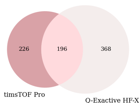
Figure 56 : Nombre de phosphopeptides identifiés dans 3/3 réplicas par les deux instruments.
