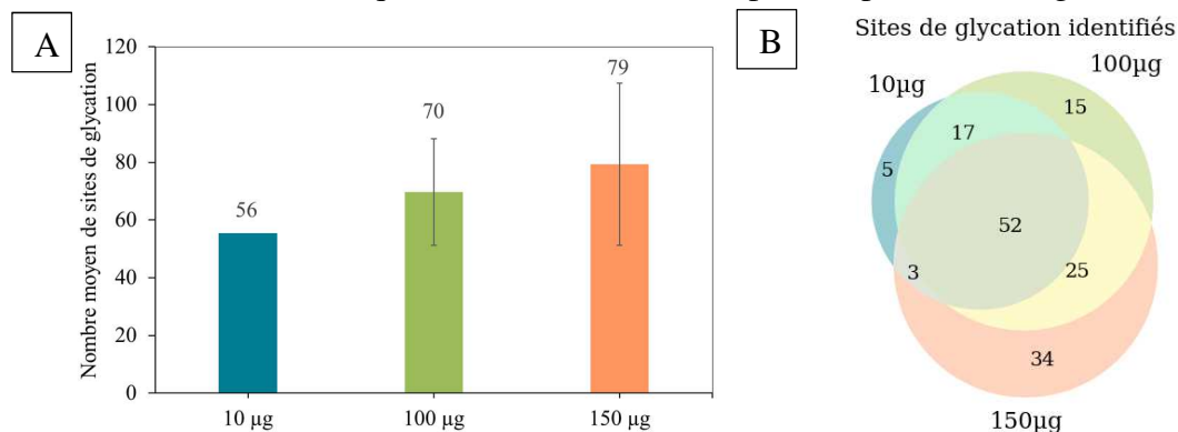
Figure 108 : Nombre moyen de sites de glycation identifiés avec le dépôt de 10 \mu\text{g} (N=2), 100 \mu\text{g} (N=3) et 150 \mu\text{g} (N=3) (A) ; Recouvrement des sites identifiés dans les 3 conditions (B).
