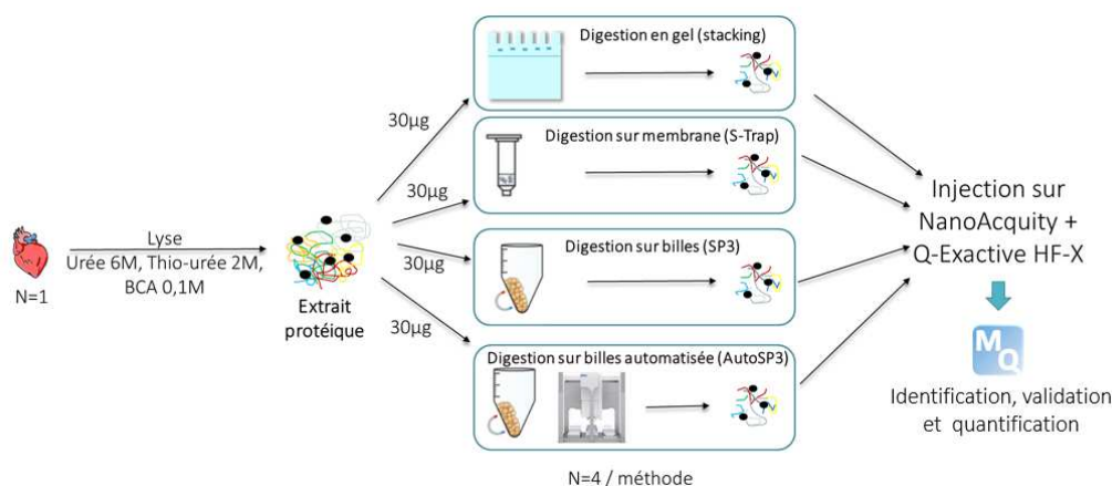
Figure 77 : Schéma analytique mis en œuvre pour comparer la digestion en gel (Stacking) aux digestions sur membrane (S-Trap), manuelle sur billes paramagnétiques (SP3) et automatisée sur bille (Auto SP3).
