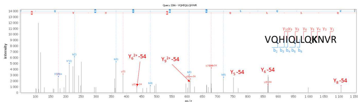
Figure 127 : Spectre de fragmentation effectué sur un Q-Orbitrap du peptide VQHIQLLQKNVR, des pertes de neutres ( 3 \times \text{H}_2\text{O} ) sont observées sur les fragments y portant la lysine glyquée.
