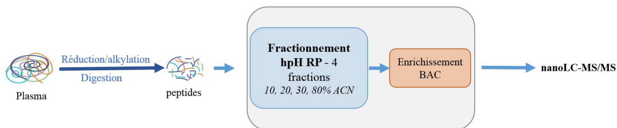
Figure 124 : Schéma expérimental du couplage entre le fractionnement hpH RP et l'enrichissement BAC.
