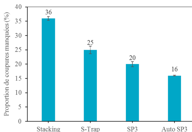
Figure 82 : Proportion de clivages manqués par la trypsine dans les différents protocoles de digestion (Stacking, S-Trap, SP3 et AutoSP3).
