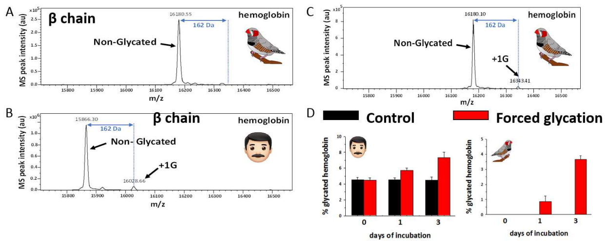
Figure 88 : Glycation de l'hémoglobine du diamant mandarin et de l'humain : spectre déconvolué de la chaîne bêta de l'hémoglobine du diamant mandarin in vivo (A) ; spectre déconvolué de la chaîne bêta de l'hémoglobine humaine in vivo (B) ; spectre déconvolué de la chaîne bêta de l'hémoglobine du diamant mandarin glyquée in vitro (C) ; proportion d'hémoglobine glyquée au cours du temps chez l'homme et le diamant mandarin dans un milieu avec (forced glycation) ou sans (control) glucose (D).
