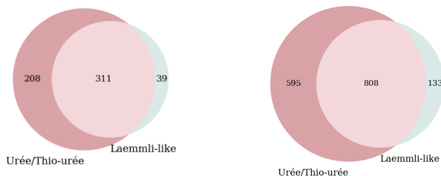
Figure 51 : Diagramme de Venn des phosphoprotéines et des phosphopeptides identifiés à partir des deux extractions réalisées : urée/thio-urée et Laemmli-like.
