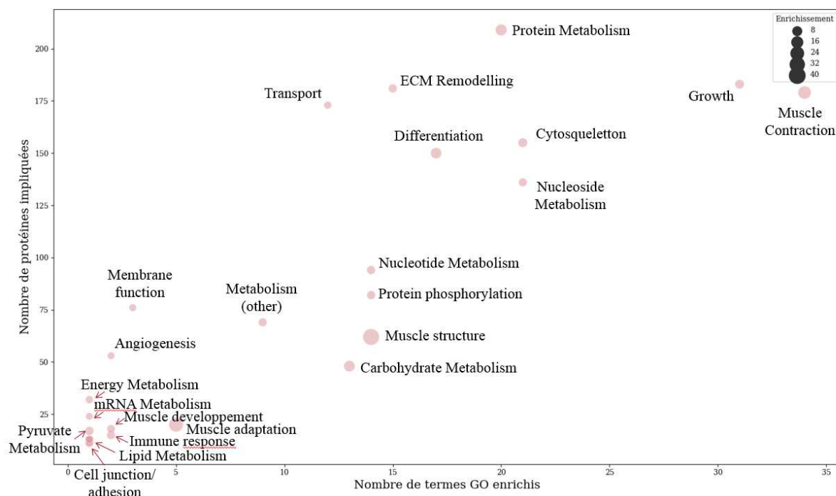
Figure 75 : Résultats du calcul d'enrichissement en annotations fonctionnelles sur les protéines portant un phosphosite dont l'abondance varie différemment entre la phase hibernante et la phase active ; ECM = matrice extracellulaire.
