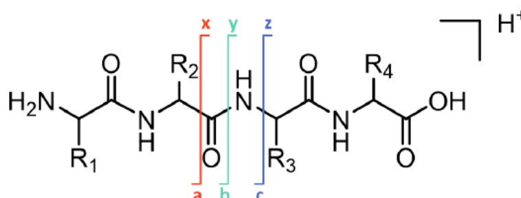
Figure 12 : Ions obtenus après fragmentation comme définis par la nomenclature de Biemann. Il existe six types d'ions : a, b, c en N-ter et x, y, z en C-ter.
