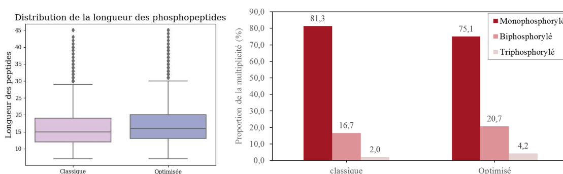
Figure 68 : Distribution de la longueur des peptides phosphorylés et du nombre de phosphorylations portés par peptides issus des identifications avec les deux méthodes MS.
