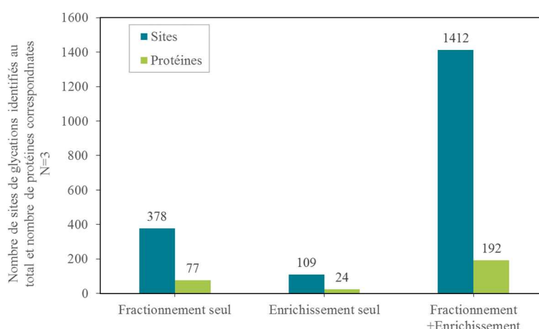
Figure 125 : Nombre total de sites de glycation identifiés dans les trois répliques des échantillons uniquement fractionnés, uniquement enrichis et fractionnés + enrichis analysés sur le Q-Exactive Plus et le nombre de protéines glyquées correspondantes.
