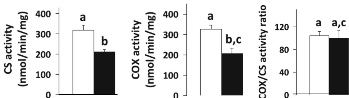
Figure 41 : Activité du cycle de Krebs (CS) et de la respiration mitochondriale (COX) et du ratio COX/CS en été (blanc) et en hiver (noir).
