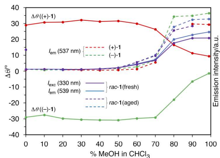
Figure 6. Evolution, en fonction du pourcentage de MeOH dans le chloroforme, du dichroïsme circulaire \Delta\theta , et de l'intensité d'émission vers 540 nm de solutions 10^{-5} M du complexe 1 sous forme énantiomériquement pure ((+)- 1 et (-)- 1 ) et racémique.
