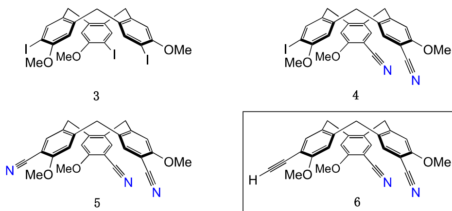
Figure 9. Structures du cyclotribenzylène-cible 6 (en encadré), de ses précurseurs 3 et 4 , et du sous-produit 5 .
