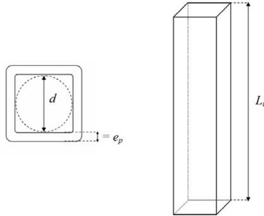
FIG. 2.1 – Schéma des tubes capillaires carrés utilisés, d est le diamètre interne (arrêté interne), e_p est l'épaisseur de paroi et L_t est la longueur du tube.
