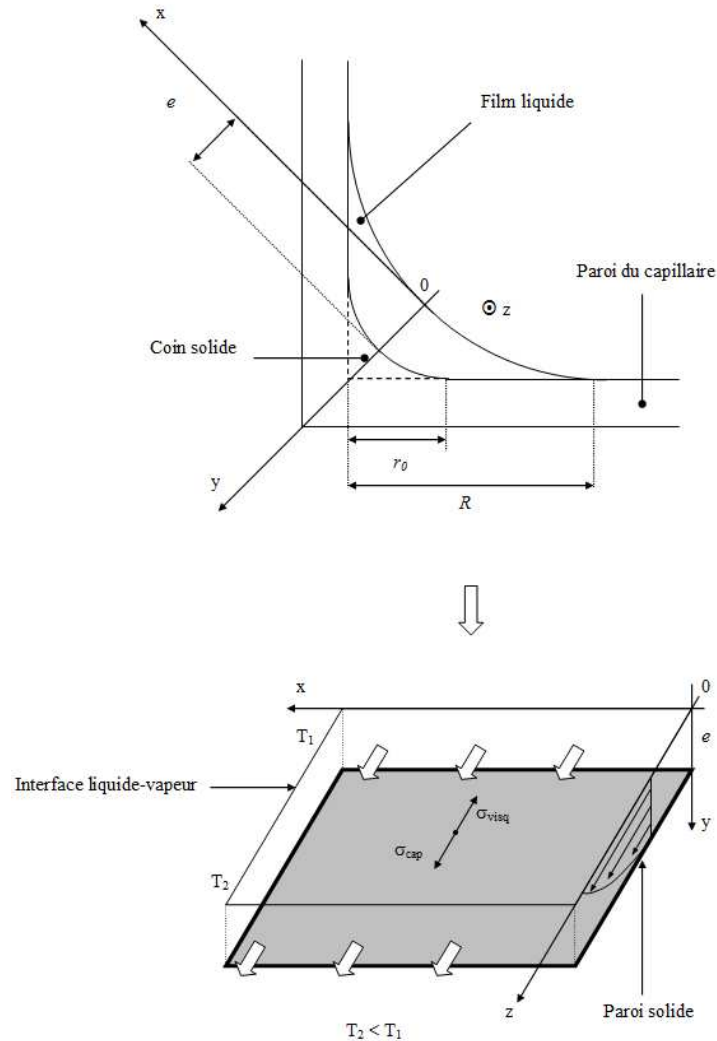
FIG. 5.18 – Schéma de la situation équivalente en film plan
