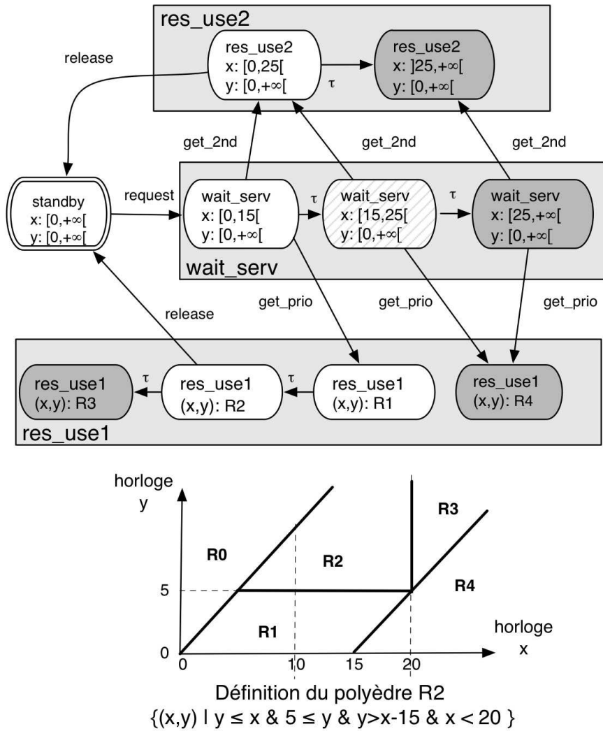
FIG. 3.3: Graphe représentant une abstraction temporelle forte de l'automate du serveur.
