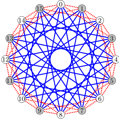
Figure 3.5. B_{16;5}
