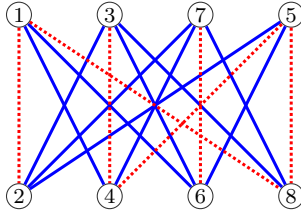
Figure 3.12. \hat{B}_{16;5}^s
