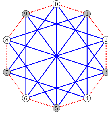
Figure 3.6. B_{10;3}
