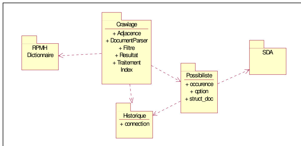
Figure 5.15 : Diagramme de classes générale de deux modules de crawlage et de tri
