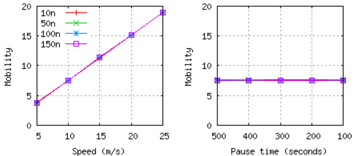
FIG. 5.1 – Mobilité de modèle Manhattan
