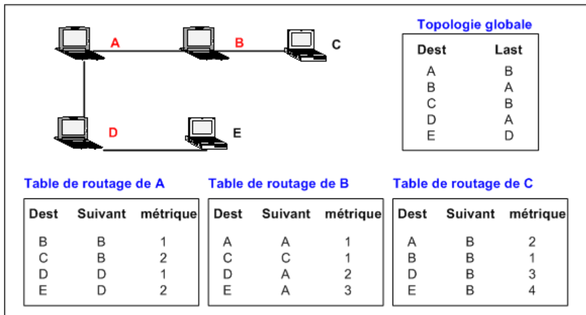
FIG. 4.1 – Exemple de routage OLSR.
