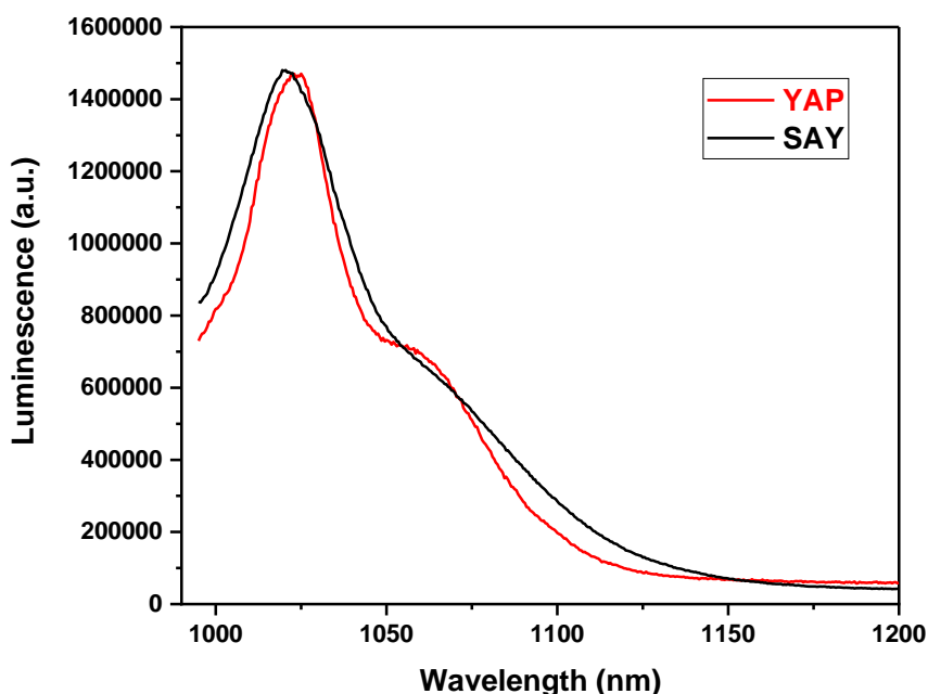
Figure 57 : Spectres d'émission des ions Yb 3+ de l'échantillon SAY (courbe noire) et YAP (courbe rouge).
