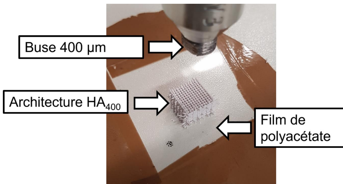
Figure 83 : Architecture HA 400 après extrusion
