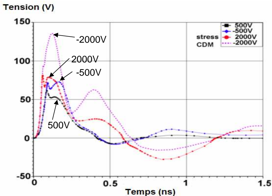
Figure 2-24 : Les tensions maximums sur les grilles des MOS M0 et M1 pour différents niveaux de tension de charge CDM simulés par TCAD-ISE en mode mixte.
