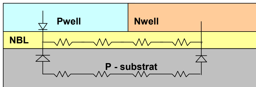
Figure 3-22 : Modélisation des diodes parasites.
