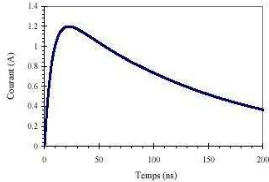
Figure 1-16: Courant de décharge du modèle HBM.
