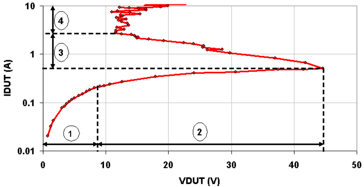
Figure 3-9 : Courbe I(V) typique sur une résistance Nwell de 5\mu\text{m} (CMOS_45nm) de l'injection faible à l'injection ultra forte après la mesure vf-TLP 2,5ns.
