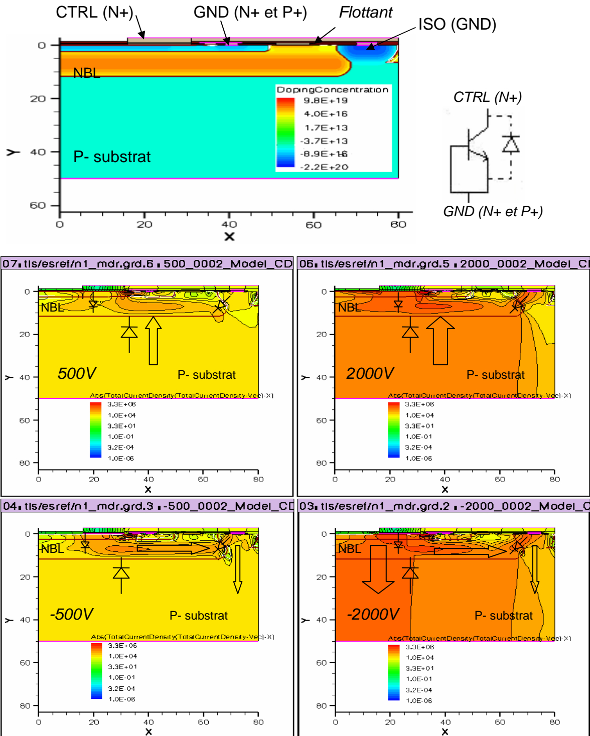
Figure 2-25 : Les densités de courant aux moments où le courant de décharge maximal pour différents niveaux de tension de charge CDM simulées par TCAD-ISE en mode mixte.
