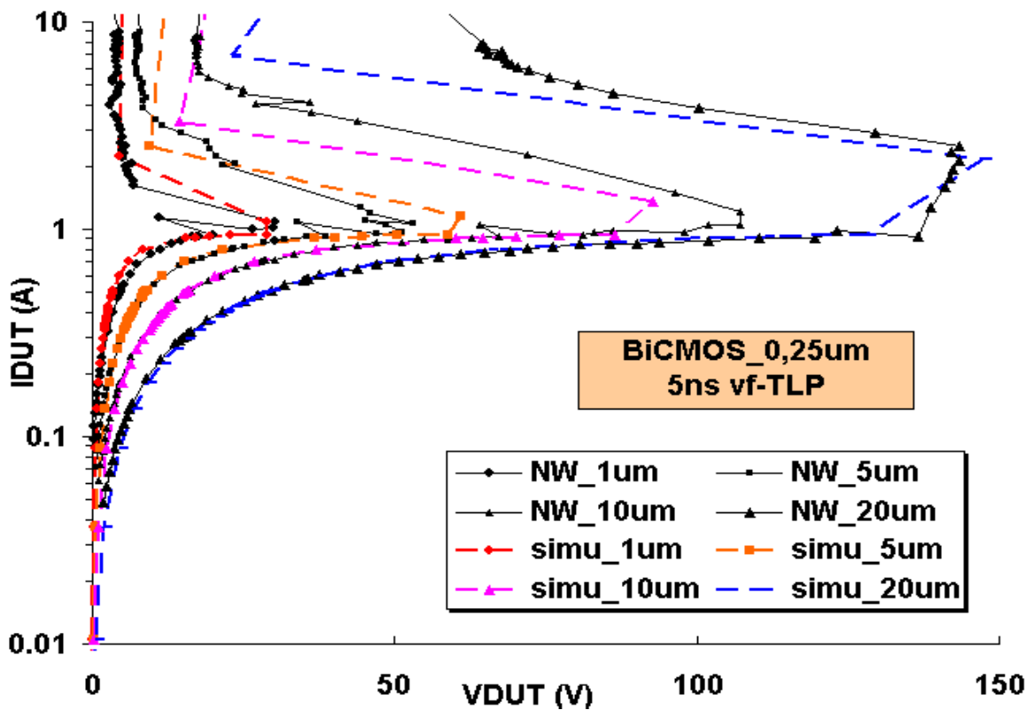
Figure 3-19 : Résultats des mesures et modèles des résistances de type N pour la technologie BiCMOS_0,25 \mu m en vf-TLP de 5ns.
