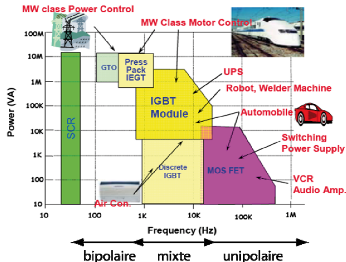
Figure I-1 : champs d'application des composants de puissance en 2005, d'après [1]
