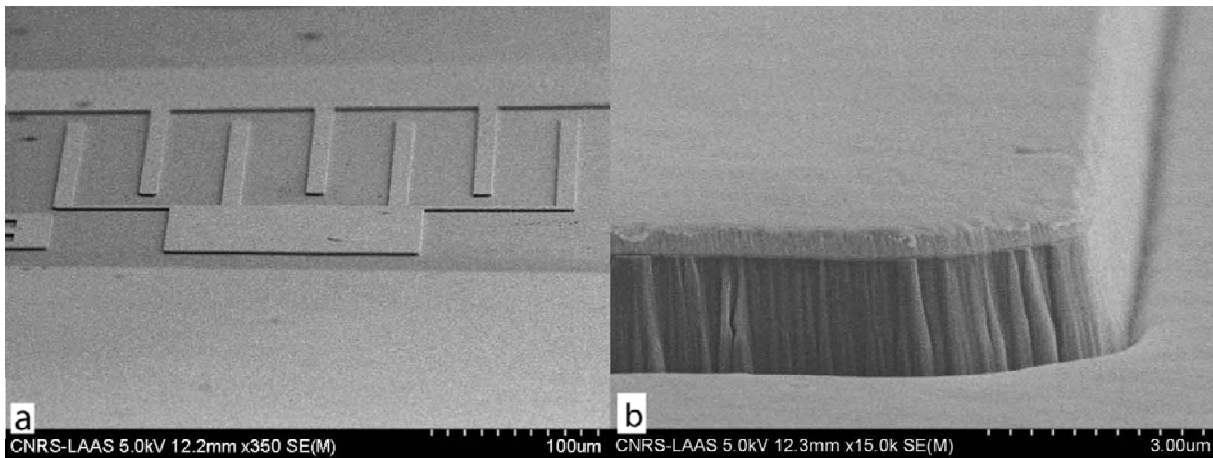
Figure III-33 : photographie MEB de l'échantillon après une gravure oxygène de 1,5 µm de profondeur. Le masque de gravure est encore en place a) motif MSM réalisé par gravure O 2 b) détail du motif
