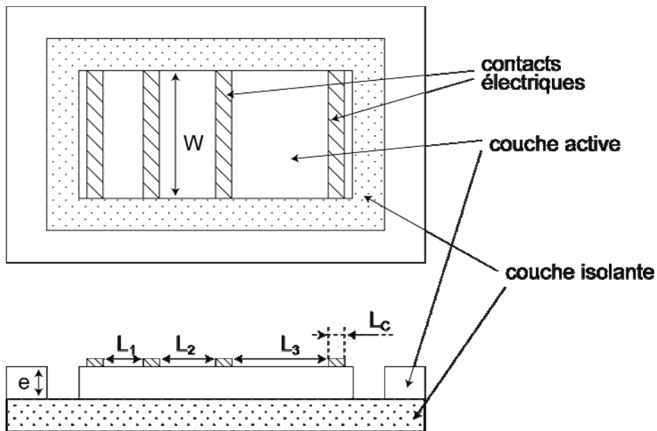
Figure III-18 : schéma d'un motif de test classique
