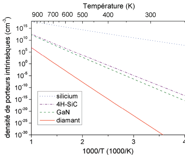
Figure I-8 : variation de la densité de porteurs intrinsèques de différents matériaux en fonction de la température
