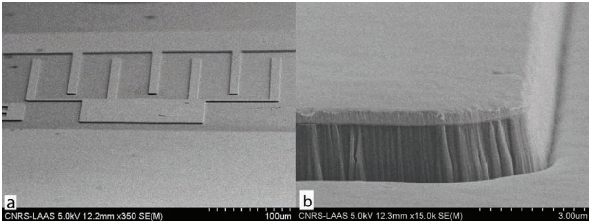
Figure III-33 : photographie MEB de l'échantillon après une gravure oxygène de 1,5 \mu\text{m} de profondeur. Le masque de gravure est encore en place a) motif MSM réalisé par gravure \text{O}_2 b) détail du motif
