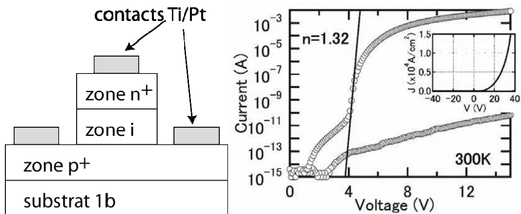
Figure II-13 : schéma en coupe de la diode pin en diamant et caractéristiques directes et inverses associées à 300 K [37]
