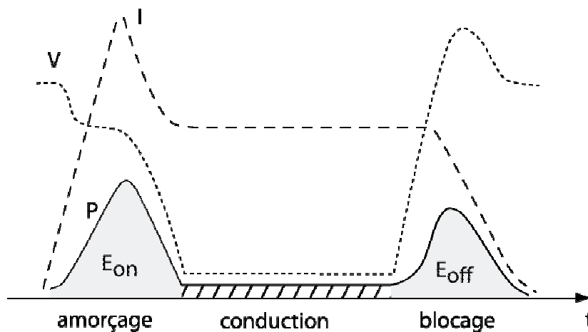
Figure I-5 : puissance dissipée dans un composant de puissance en commutation en fonction du temps
