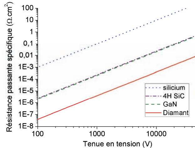
Figure IV-3 : résistance spécifique à l'état passant en fonction de la tenue en tension calculées d'après l'Équation IV-3 pour le silicium, le SiC 4H, le GaN et le diamant à 300 K
