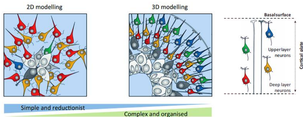
Figure 36. Modélisation de la corticogenèse in vitro 2D et 3D (van den Aemele et al., 2014)
