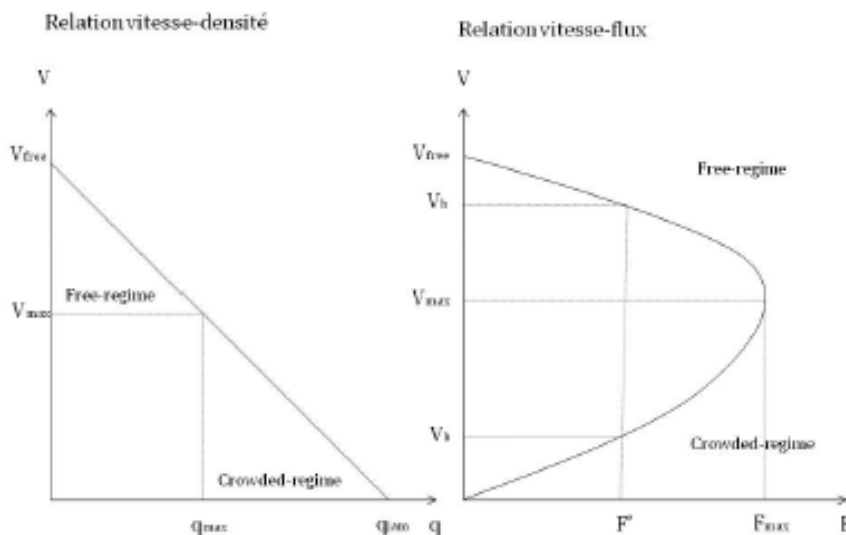
Graphique 21: relation vitesse concentration de véhicules.
