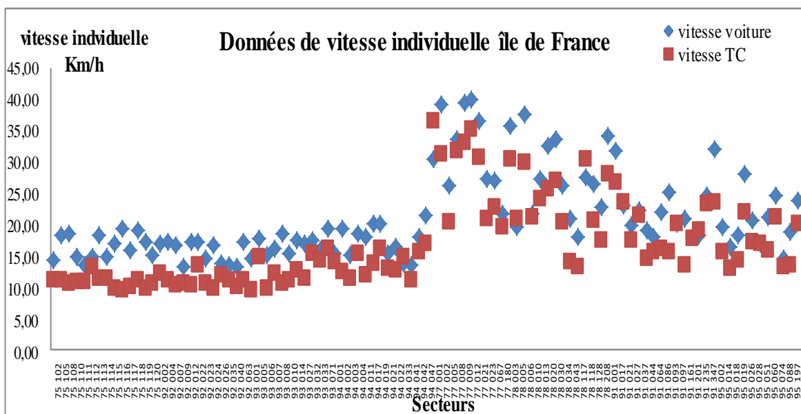
Graphique 47: données de vitesses de déplacement par secteur
