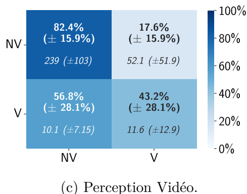
FIGURE 5.15 – Matrice de confusion en fonction de la perception des violences pour l’architecture combinant les signaux par concaténation à un niveau moyen. Résultats, en pourcentage et nombre d’instances, obtenus sur 100 répartitions avec "NV" pour les exemples sans violences et "V" les exemples avec violences. Entre parenthèse : variance en pourcentage et en nombre d’instances.
