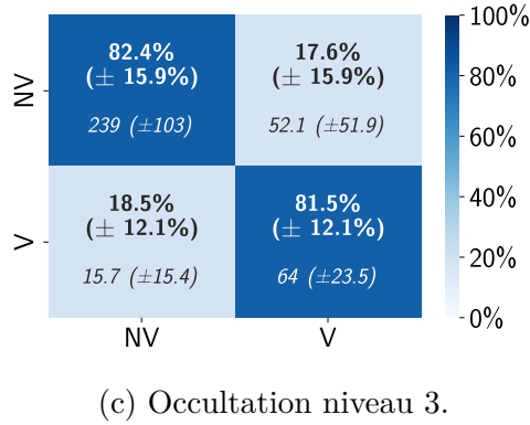
FIGURE 5.17 – Matrice de confusion en fonction du degré d’occultation pour une architecture combinant les signaux par concaténation à un niveau moyen. Résultats, en pourcentage et nombre d’instances, sur 100 répartitions avec "NV" pour les exemples sans violences et "V" les exemples avec violences. Entre parenthèse : variance en pourcentage et en nombre d’instances.
