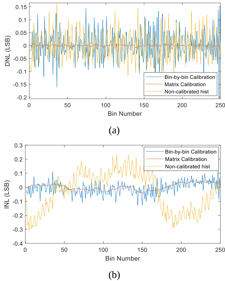
Figure 5. Valeurs de DNL et de INL du TDC asynchrone avant et après appliquer la calibration bin-par-bin et la calibration matricielle : (a) valeurs de DNL, (b) valeurs de INL.
