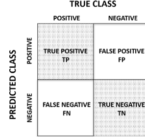
Fig. 6. Confusion matrix.
