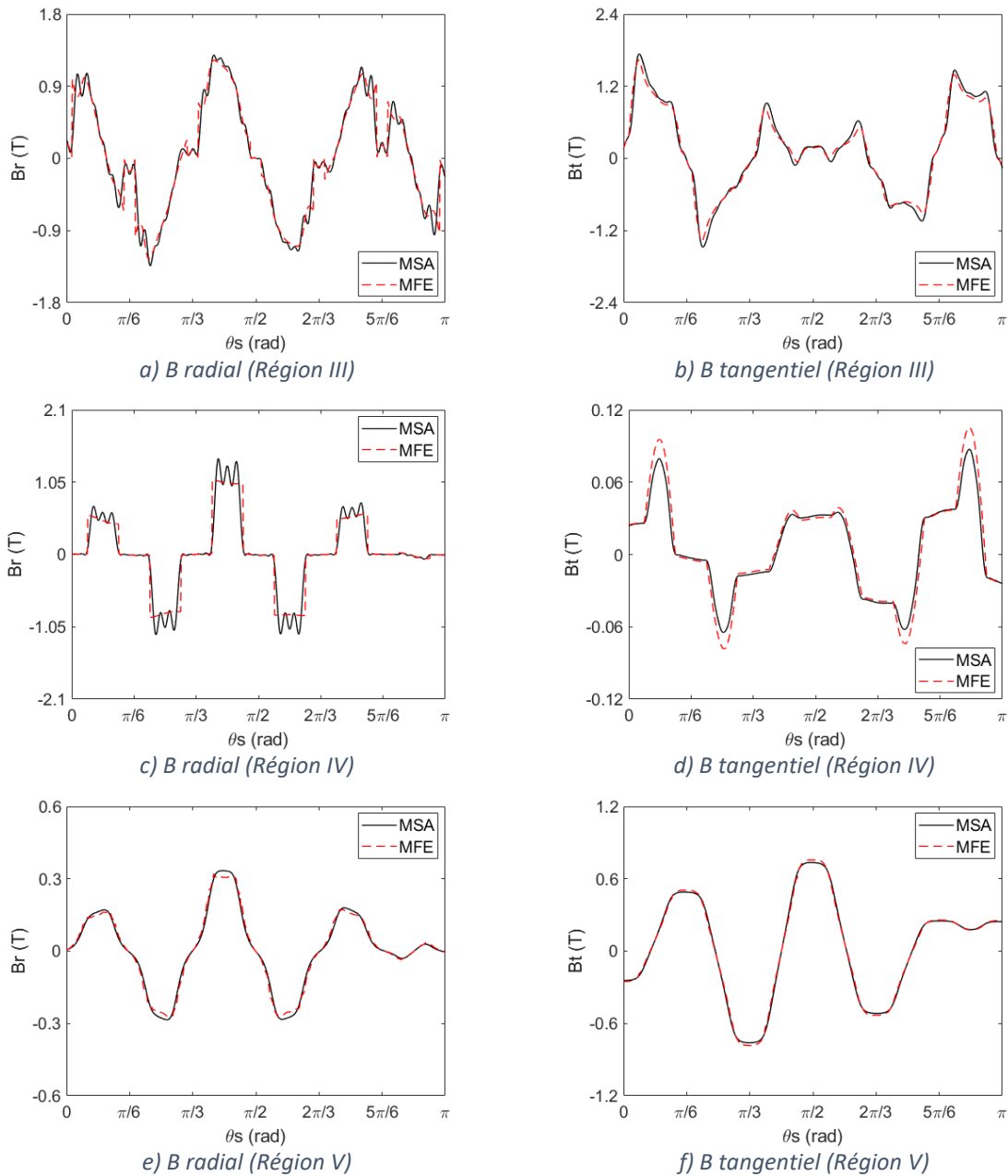
Figure 2.18 - Comparaison entre MSA et MEF des composantes B_r et B_t au rayon moyen des Régions III, IV et V pour \mu r = 90,92 dans le stator ( I_{max} = 20 A, 1500 rpm et \theta = 0^\circ ).
