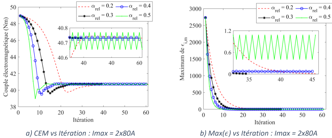
Figure 2.25 - Évolution de la convergence de la méthode Relaxation dans le cas saturé ( I_{max} = 2x80A ).
