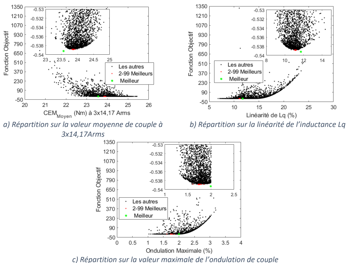
Figure 4.37 - Répartition des valeurs de fonction Objectif selon les valeurs de contraintes, pour la 2 ème étape de l'optimisation complète de la machine Halbach Continu à 10 pôles.
