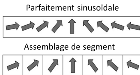
Figure 1.10 - Différents type de fabrication de la configuration Halbach.
