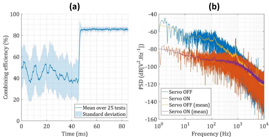
Figure 59 : Comportement dynamique de l'asservissement par la méthode PIM-PR (Phase Intensity Mapping with Phase Retrieval). (a) Qualité de phasage moyenne mesurée sur 25 cycles de mise en phase et (b) DSP correspondantes en boucle ouverte et fermée et leur moyenne mobile. Les courbes se croisent à environ 2 kHz. Résultats présentés dans [119].
