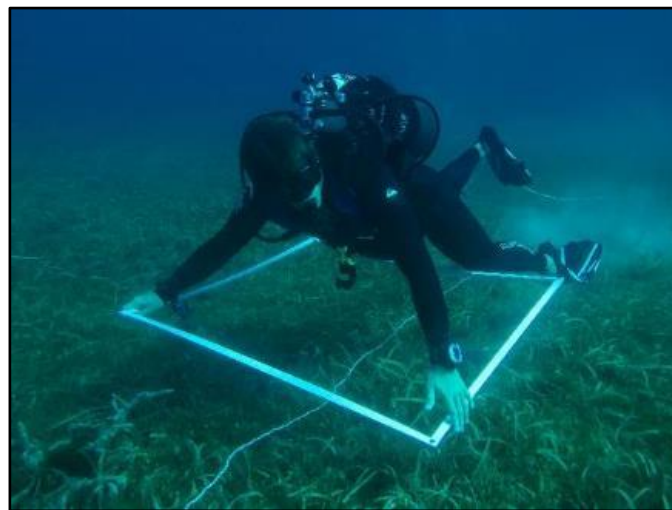
Figure 3-10. Détermination du pourcentage de recouvrement du sol par les plantes marines par un plongeur utilisant un quadrat. Crédit photo : CNRS.
