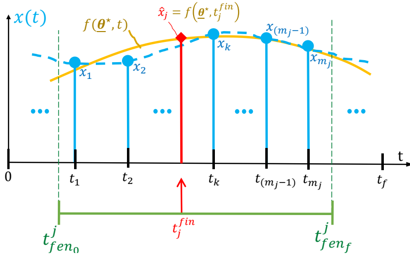
FIG. 3.5 – Reconstruction du point associé à la fenêtre, \hat{x}_j = f(\underline{\theta}^*, t_j^{fin})
