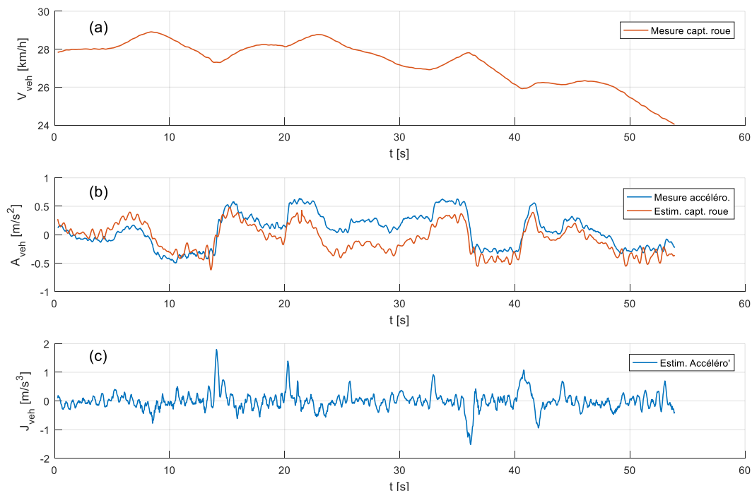
FIG. 3.14 – Estimation des signaux d'accélération et d'à-coup. (a) « mesure » de vitesse à partir des capteurs des roues; (b) accélération, mesurée et estimée (c) estimation de l'à-coup à partir du signal de l'accéléromètre
