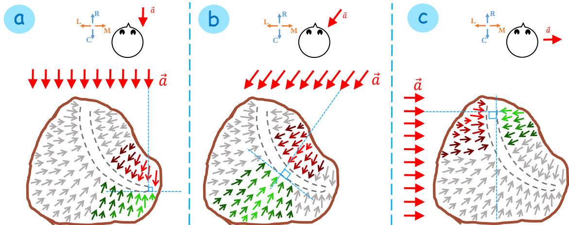
FIG. 1.8 – Polarisation directionnelle de la macula ; les flèches vertes correspondent aux cellules excitées, les rouges aux cellules inhibées et les grises aux cellules au repos. Les flèches les plus claires sont celles le plus fortement activées. (a) accélération longitudinale ; (b) accélération en biais ; (c) accélération latérale.
