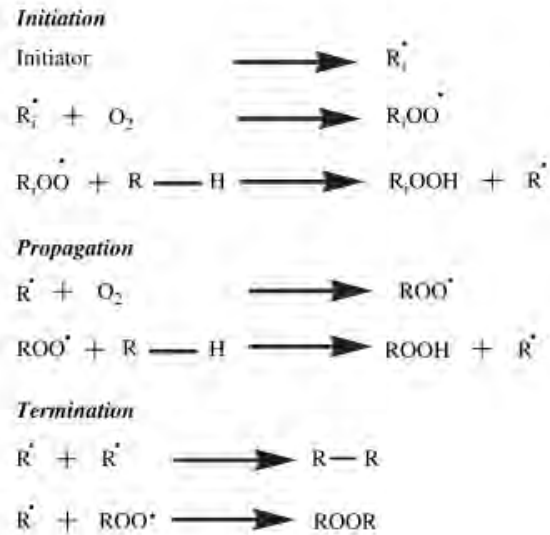
Figure 2. Schéma du processus de photodégradation, montrant les 3 étapes du processus : Initiation, propagation et terminion. 37
