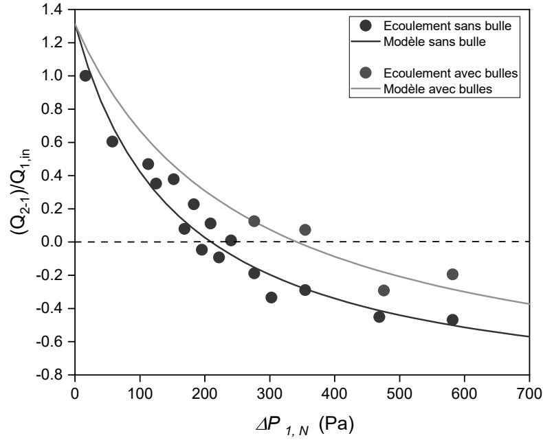
Figure 11.6 Débit normalisé dans le passage reliant les deux puces, avec et sans bulles, en fonction de la perte de charge estimée dans l'aiguille de sortie de la puce inférieure pour Q_{in} = 1 mL/min. Les lignes représentent les prévisions par l'équation 11.5 sans (bleu) et avec (vert) bulles.
