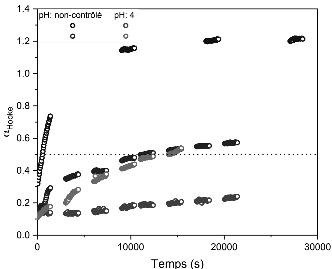
Figure 7.13 Evolution de \alpha au cours de quatre expériences en fonction du temps pour différents pH : [\text{NaPSS}] = 4,8 \text{ mM} , [\text{NaCl}] = 0,15 \text{ M} , f = 0,02 \text{ Hz} , amplitude : 10 %.
