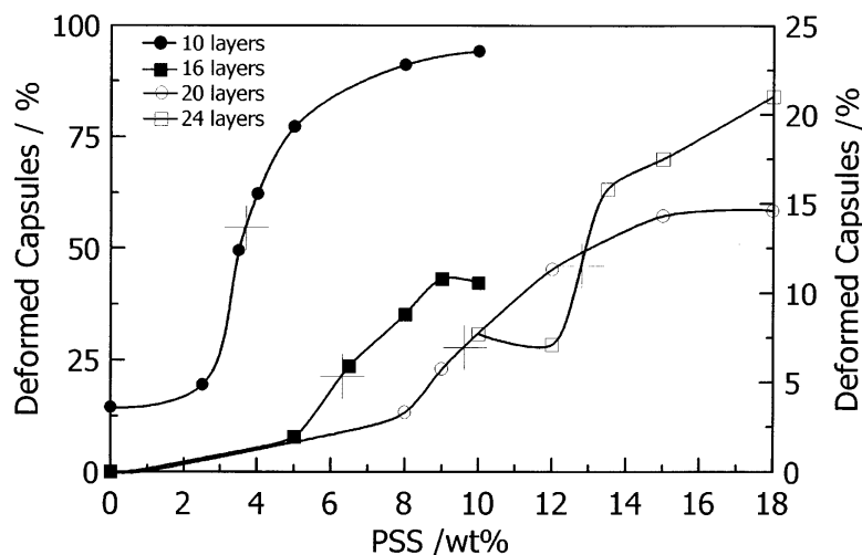
Figure 2.17 Pourcentage de capsules PSS/PAH déformées en fonction de la concentration en PSS en solution pour créer une pression osmotique (rayon des capsules : 2\ \mu\text{m} . Nombre de couches indiqué dans la légende. L'axe de gauche est utilisé pour les symboles fermés et l'axe de droite pour les symboles ouverts. Les croix indiquent les points de transition critiques (source : Gao et al. 5 ).
