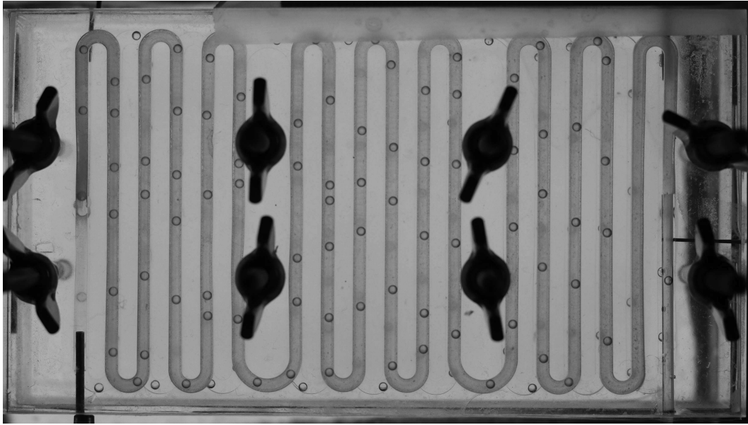
Figure 11.7 Ecoulement de bulles dans la puce inférieure. Bullage réalisé avec Q_{in} = 1 \text{ mL/mn} , P_G = 1740 \text{ Pa} (17.4 mbar) et \Delta P_{1,N} = 355 \text{ Pa} .
