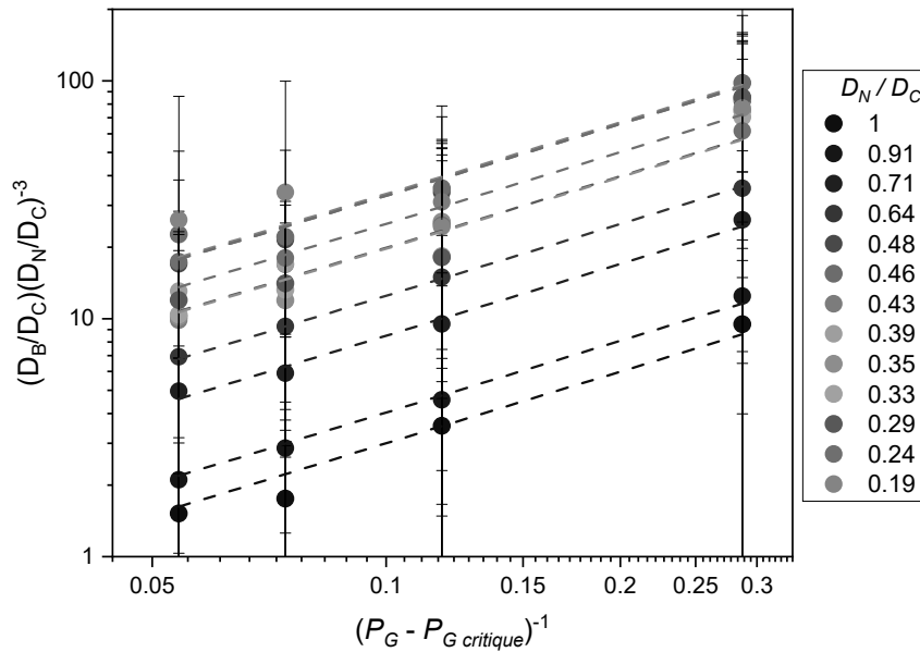
Figure 10.7 Évolution de \frac{D_B}{D_C} \left( \frac{D_N}{D_C} \right)^{-3} avec (P_G - P_{G,crit})^{-1} pour différentes valeurs de \frac{D_N}{D_C} dans une solution de NaPSS avec Q_L = 1 mL/mn. Les lignes sont des ajustements linéaires avec des droites de pente 1.
