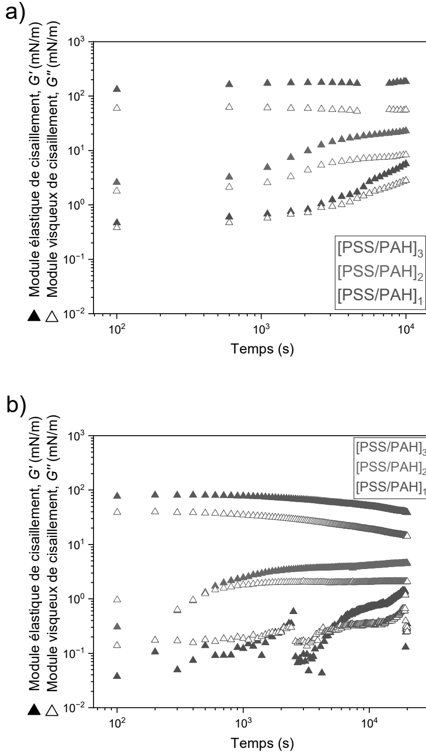
Figure 9.9 Effet du nombre de couches de polyelectrolytes adsorbées sur l'évolution temporelle de G' et G'' . (a) Expérience 1, f = 0,01 Hz, A_0 = 0,08\% . (b) Expérience 2, f = 0,01 Hz, A_0 = 0,3\% .
