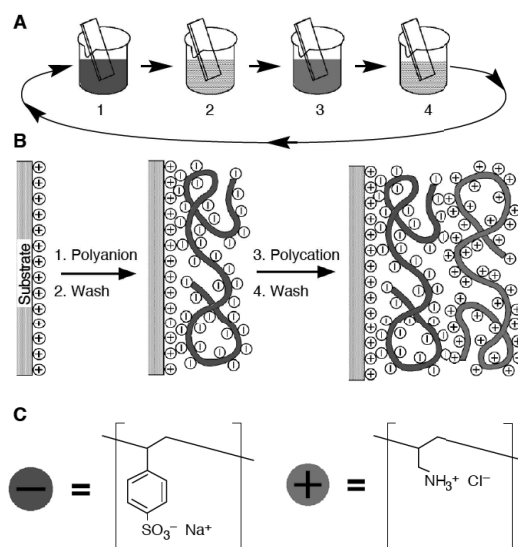
Figure 2.14 (A) Schéma de la construction d'un film multicouches par trempage. Les étapes 1 et 3 représentent l'adsorption d'un polyanion et d'un polycation, respectivement, et les étapes 2 et 4 sont des étapes de lavage. Les quatre étapes sont la séquence de construction de base pour l'architecture de film la plus simple, (A/B) _n . (B) Schéma moléculaire simplifié des deux premières étapes de l'adsorption, décrivant le dépôt d'un film à partir d'un substrat chargé positivement. Les contre-ions sont omis pour plus de clarté. La conformation et l'interpénétration des couches de polyélectrolytes sont idéalisées pour représenter l'inversion de la charge de surface à chaque étape de l'adsorption. (C) Structures chimiques de deux polyélectrolytes typiques, la poly(styrène sulfonate) et la poly(allylamine hydrochloride) (source : Decher 1 ).
