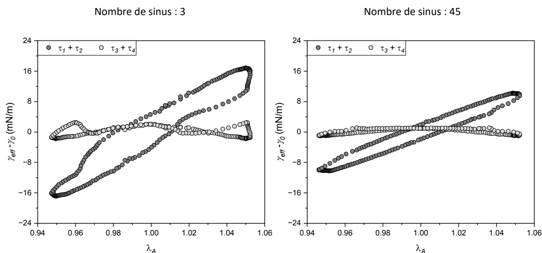
Figure 8.15 Comparaison des contraintes \tau_1 + \tau_2 et \tau_3 + \tau_4 après l'adsorption de 6 couches ([PSS/PAH] 3 ) pour les expériences où l'interface subit 3 cycles (à gauche) ou 45 cycles (à droite) de déformations sinusoïdales après l'adsorption.
