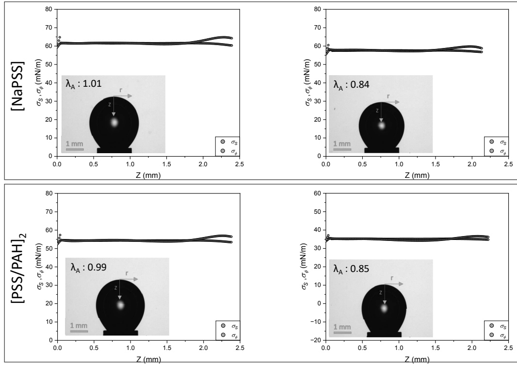
Figure 8.17 Evolution des contraintes \sigma_s et \sigma_\phi le long du profil droit d'une bulle de gaz dans l'eau saline ( [NaCl] = 0,15 M) après l'adsorption d'une couche de NaPSS(en haut) ou de quatre couches de polyélectrolytes ( [PSS/PAH]_2 ) (en bas).
