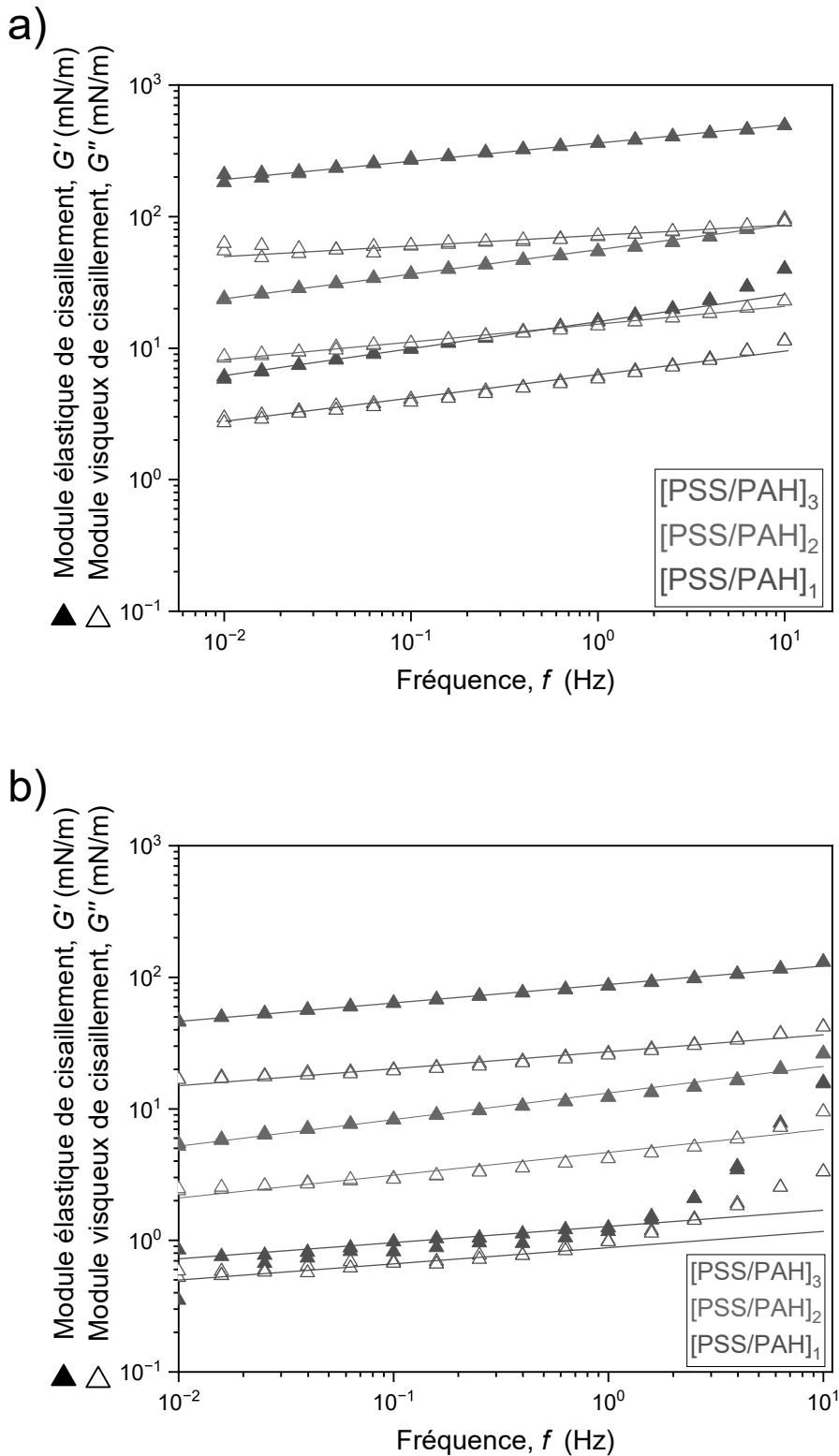
Figure 9.10 Evolution de G' et G'' avec la variation de fréquence de mesure et du nombre de couches de polyelectrolytes adsorbées à l'interface (amplitude : 0,08 %). (a) Expérience 1, pré-déformée à une amplitude de 0,08 % pendant le premier balayage temporel. (b) Expérience 2, pré-déformée à une amplitude de 0,3 % pendant le premier balayage temporel.
