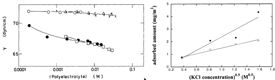
Figure 2.3 (à gauche) Evolution de la tension de surface avec la concentration pour NaPSS (○), \text{Et}_4\text{NPSS} (×), \text{Pr}_4\text{NPSS} (□), \text{Bu}_4\text{NPSS} (●) (source : Okubo 44 ). (à droite) Variation de l'excès de surface \Gamma avec la racine carrée de la concentration en KCl pour deux poids moléculaires de NaPSS M_w = 56\,000 (○) et M_w = 1\,150\,000 (●) (source : Yim et al. 45 ).
