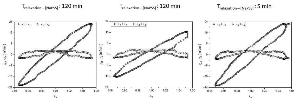
Figure 8.14 Comparaison des contraintes \tau_1 + \tau_2 et \tau_3 + \tau_4 après l'adsorption de 6 couches ([PSS/PAH] 3 ) pour les 3 expériences où l'interface subit 10 cycles de déformations sinusoïdales après l'adsorption.
