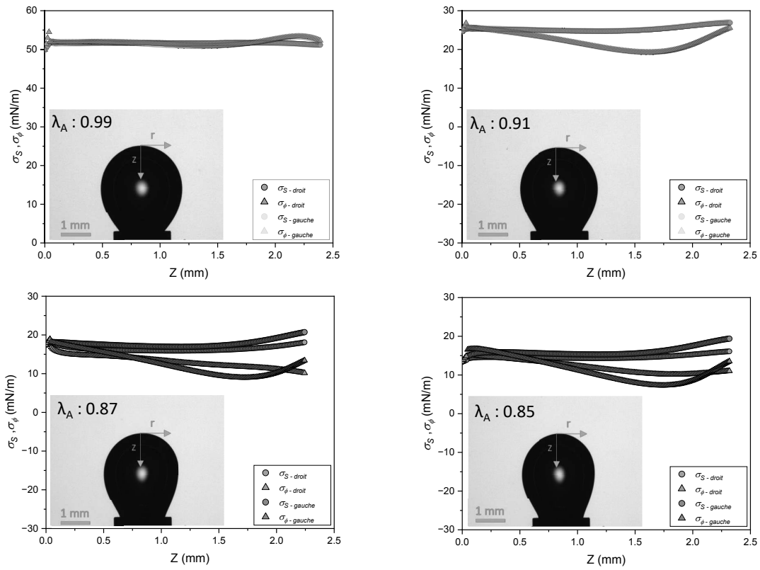
Figure 8.18 Evolution des contraintes \sigma_s et \sigma_\phi le long de chaque profil d'une bulle de gaz dans l'eau saline ( [\text{NaCl}] = 0,15 \text{ M} ) après l'adsorption de cinq couches ( [\text{PSS}/\text{PAH}]_2\text{PSS} ) de polyélectrolytes pendant une expérience de dégonflement linéaire.
