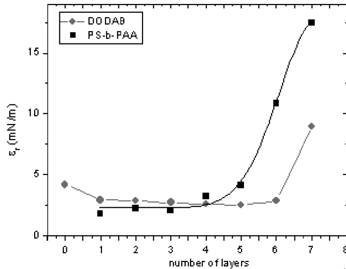
Figure 2.18 Dépendance de l'élasticité \epsilon_r au nombre de couches pour des multicouches adsorbées sur DODAB et sur PS-b-PAA à 20 °C et à une fréquence de 200 Hz (adapté de Safouane et al. 101 ).
