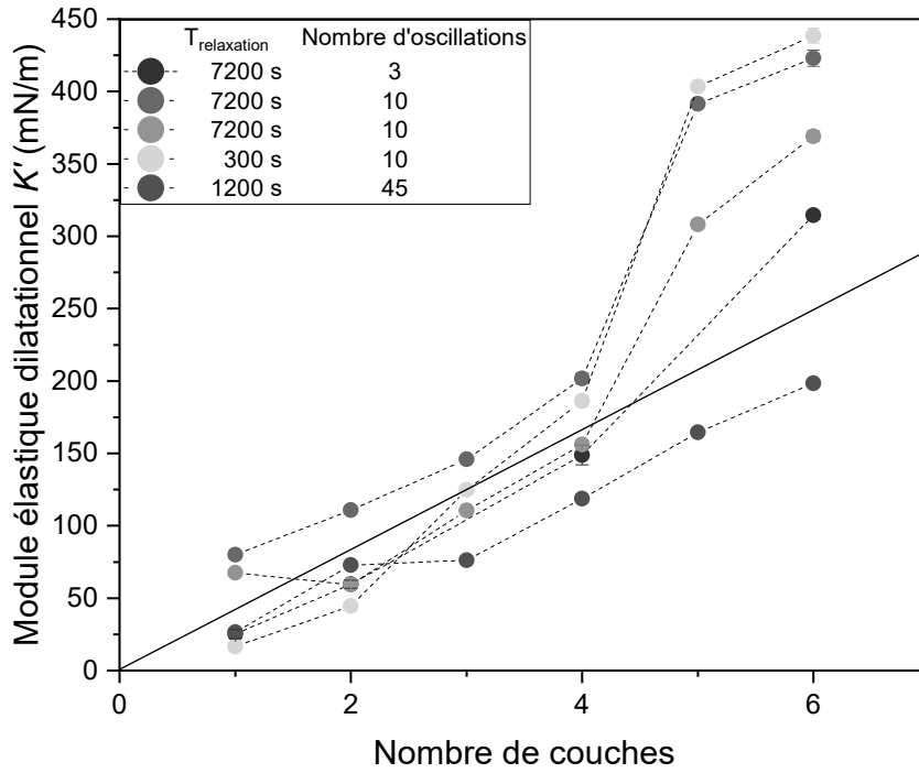
Figure 8.10 Evolution du module élastique dilatationnel interfacial K' en fonction du nombre de couches de polyélectrolytes adsorbées à l'interface. Les lignes pointillées sont des guides pour les yeux. ( f = 0,02 Hz, \lambda_0 = 5 %)
