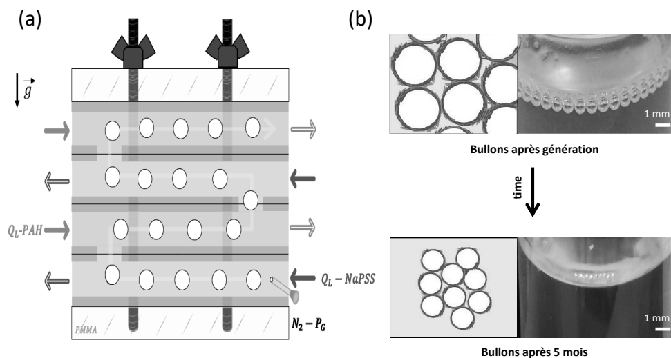
Figure 1.4 (a) Schéma du montage à 4 puces microfluidiques. (b) Évolution des bulles récoltées au cours du temps.
