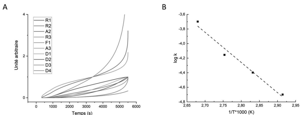
Figure 33 : Faisceau des courbes modèles pour le matériau mélamine/nitroglycérine pour une isotherme à 100°C (A), évolution \log(k) en fonction de 1/T \cdot 1000 (B)
