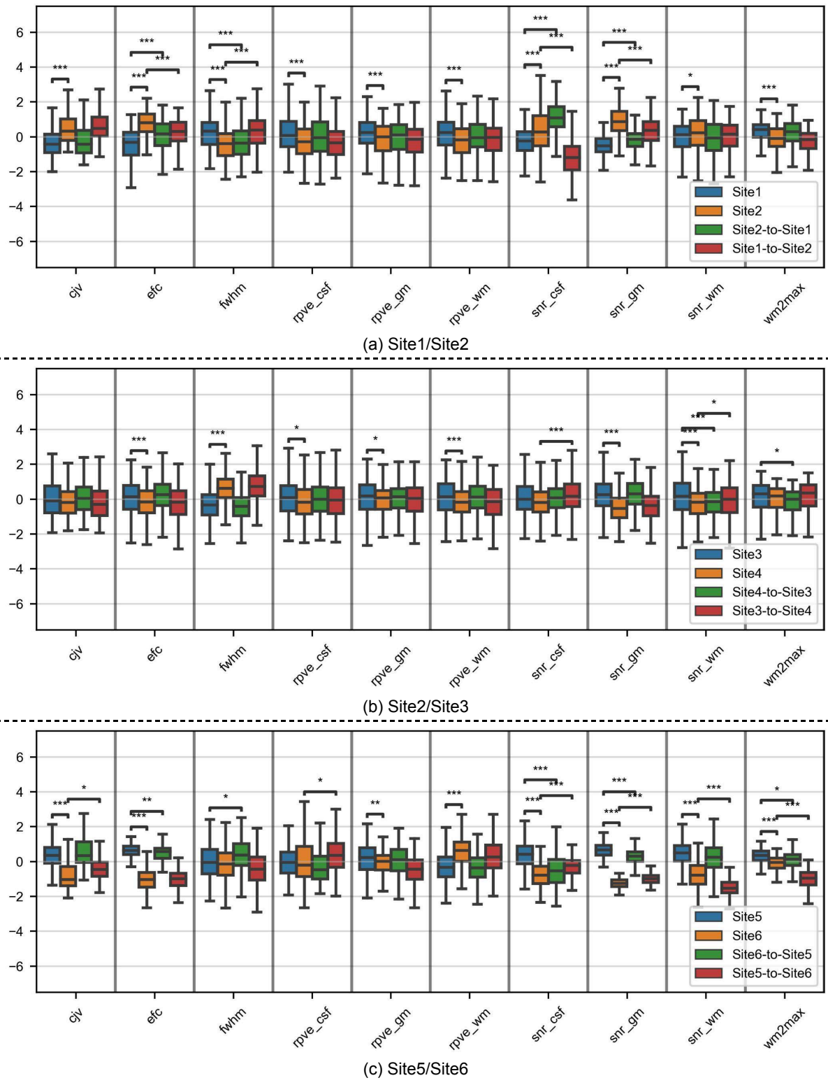
Figure 29 : Distributions des métriques de qualité d'image dans les expériences sites-appariés de la section 4. Pour chaque sous-figure et chaque métrique, l'axe de Y est un Z-score basé sur les deux ensembles d'images originales. Des astérisques indiquent des t-tests significatifs avant et après harmonisation entre les sites source et cible (* : p < 0.05 ; ** : p < 0.01 ; *** : p < 0.001 ).
