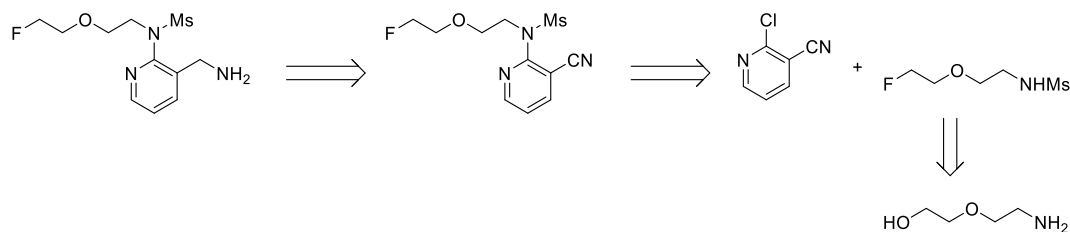
Schéma II.17: Analyse rétrosynthétique conduisant au synthon pyridine du composé PEG-FAK
