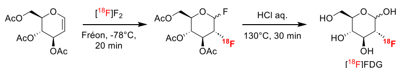
Schéma 10: Synthèse historique du [^{18}\text{F}]\text{FDG} par fluoration électrophile
