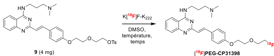
Schéma I.18: Radiomarquage au fluor-18 du composé [^{18}F]PEG-CP31398
