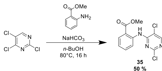
Schéma II.22: Synthèse du synthon dichloropyrimidine 35
