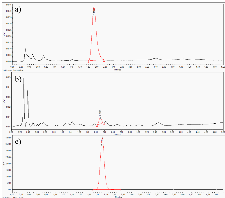
Figure III.8 Contrôle qualité du composé [^{18}\text{F}]\text{FH-SK1} réalisé par HPLC analytique sur phase inverse C18 avec détection UV (254 nm) et gamma. a) Chromatogramme UV du composé FH-SK1 de référence non radioactif ; b) Chromatogramme UV du composé [^{18}\text{F}]\text{FH-SK1} ; c) Chromatogramme gamma du composé [^{18}\text{F}]\text{FH-SK1}
