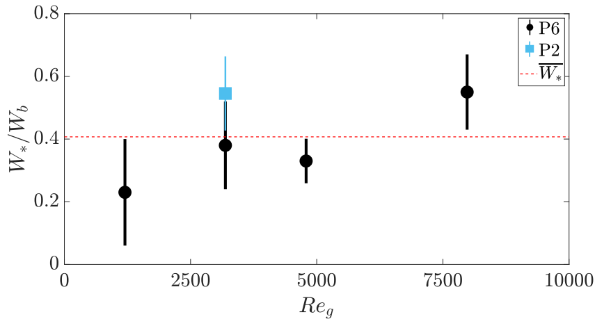
FIGURE 5.22 – Evolution de la vitesse moyenne de remontée, W_* , en fonction du forçage de grille, Re_g . La vitesse est normalisée par la vitesse de flottabilité d'un particule isolée dans un fluide au repos, W_b . La ligne pointillée rouge correspond à la valeur moyenne de W_* .
