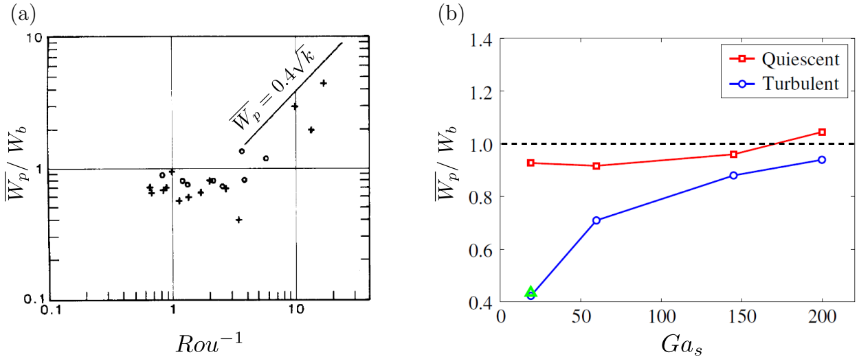
FIGURE 1.18 – (a) Vitesse moyenne de remontée d’une particule dans un écoulement turbulent, \overline{W}_p , normalisée par la vitesse de Stokes, W_b , en fonction de l’inverse du nombre de Rouse, Rou . Figure adaptée de Nielsen (1993). (b) Rapport de \overline{W}_p/W_b en fonction du nombre de Galilée, Ga_s . Figure adaptée de Fornari et al. (2016b).
