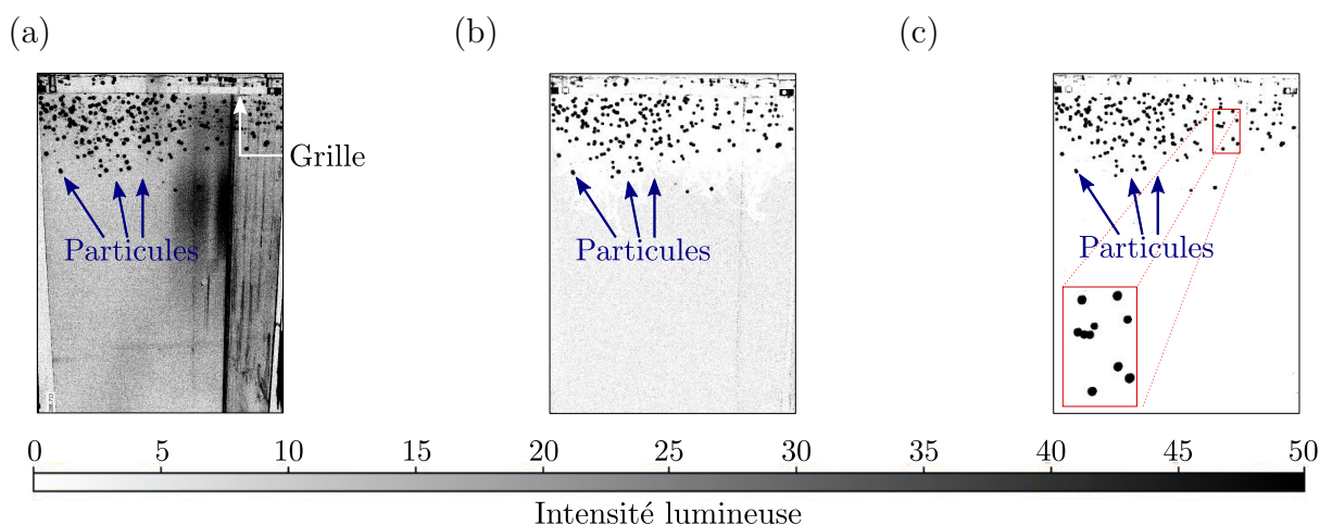
FIGURE 2.12 – Image de la caméra 1 : (a) sans pré-traitement ; (b) une fois l’image de fond soustraite et (c) une fois l’image de fond soustraite et l’intensité du fond imposée à zéro.
