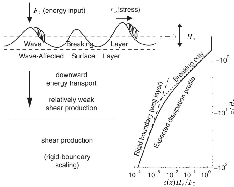
FIGURE 1.28 – Représentation schématique de la couche proche surface (" surface boundary layer " en anglais) influencée par des vagues déferlantes. \tau_w représente la contrainte du vent à l'origine de la formation des ondes de surface et \epsilon est le taux de dissipation. Figure adaptée de Gerbi et al. (2009).
