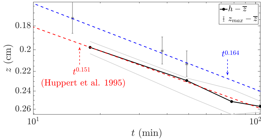
FIGURE 5.9 – Evolution temporelle de la position de l'interface, h , et de la profondeur maximale atteinte par les particules, z_{max} . Les lignes pleines grises indiquent l'épaisseur de l'interface et \bar{z} est la position moyenne de la grille.
