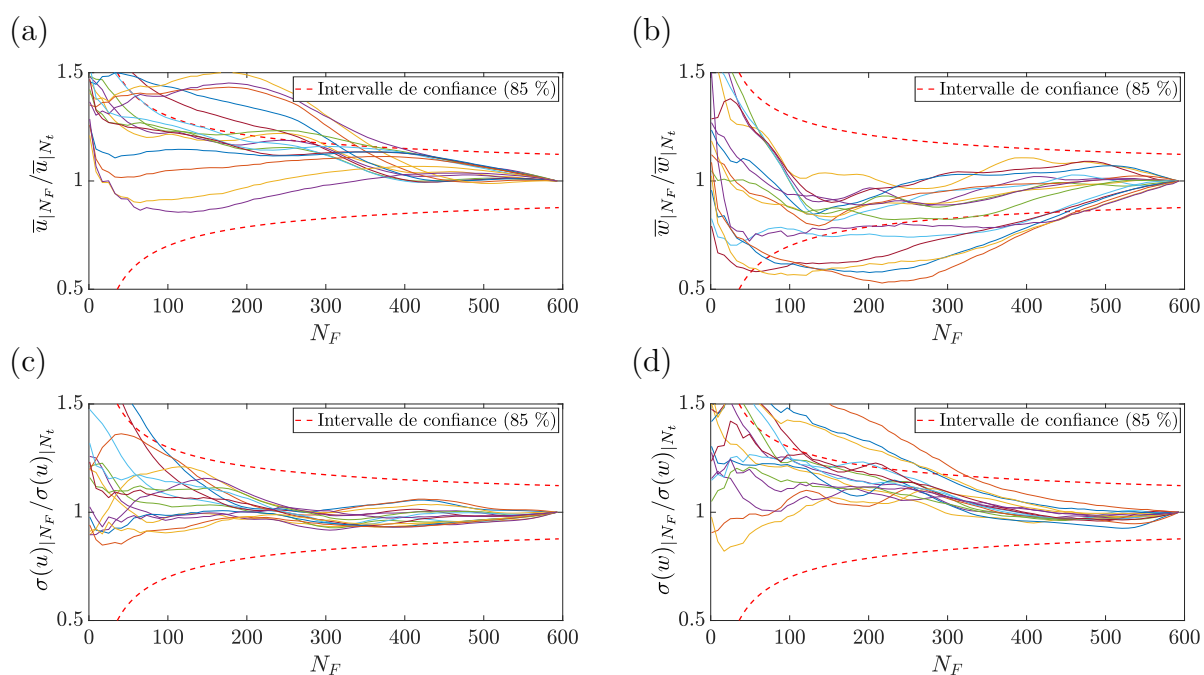
FIGURE 2.36 – Étude de la convergence statistique des mesures par PIV pour : (a) la vitesse moyenne horizontale, \bar{u} ; (b) la vitesse moyenne verticale, \bar{w} ; (c) l'écart type de la vitesse horizontale, \sigma(u) ; (d) l'écart type de la vitesse verticale, \sigma(w) . Les lignes continues correspondent aux champs de vitesses à une altitude arbitraire donnée. N_F est le nombre d'images sur lequel sont calculés la moyenne et l'écart type. N_t est le nombre total d'images.
