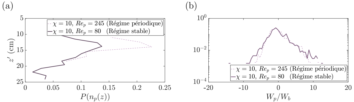
FIGURE 6.2 – (a) Probabilité de présence du disque, P(n_p(z)) , pour deux disques isolés dans une turbulence de grille oscillante avec Re_g = 7\,980 . Les disques ont des Reynolds particuliers tels que dans un fluide au repos leur régime de sédimentation est soit stable, soit périodique. (a) Pdf de la composante verticale de la vitesse, W_p , normalisée par celle dans un fluide au repos des deux disques isolés.
