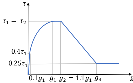
FIGURE 2.7 – Courbe enveloppe initiale de la loi d’adhérence de [Murcia-Delso et al. , 2011].
