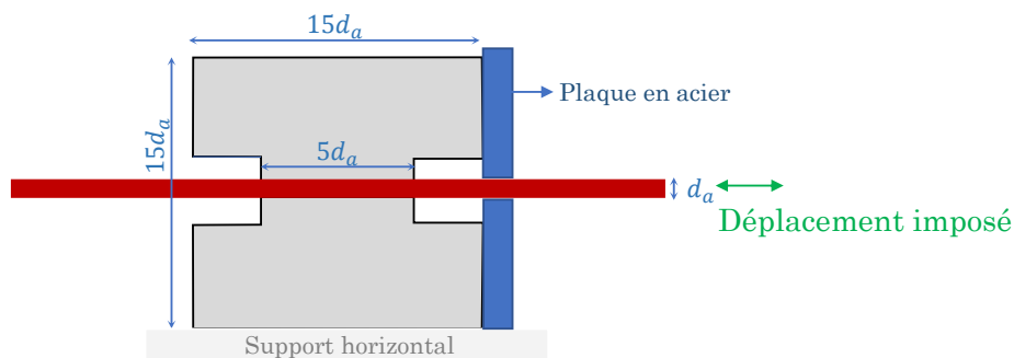
FIGURE 3.6 – Principe de l’essai de pull-out de [Torre-Casanova, 2012].
