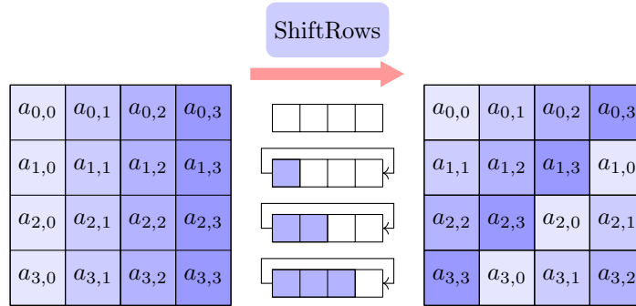
FIGURE 1.9 – Sous-fonction ShiftRows .
