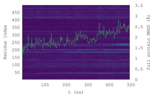
(b) Traj. 7
