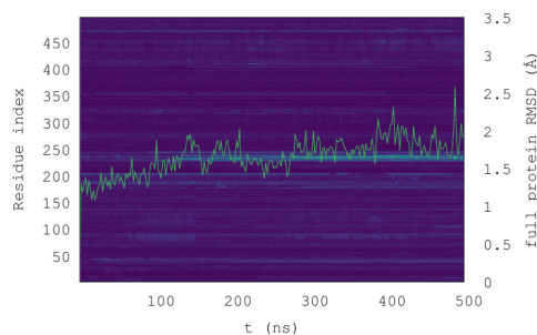
(d) Traj. 9
