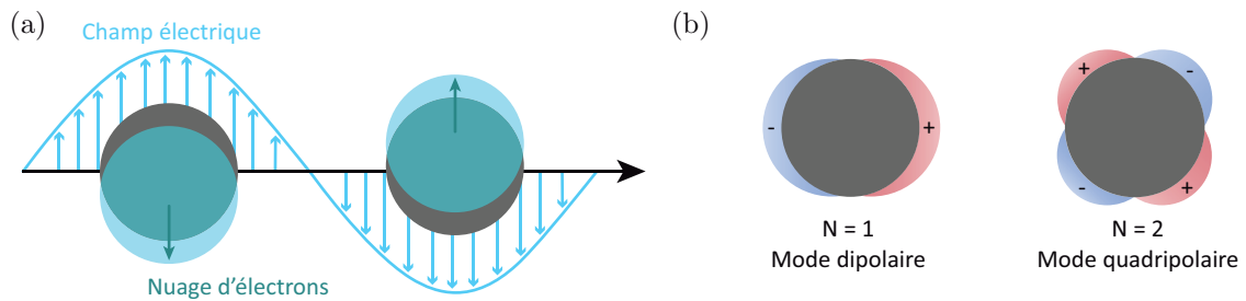
FIGURE 1.36 – (a) Représentation de l'oscillation collective du nuage d'électrons d'une nanoparticule sphérique soumise à un champ électromagnétique \mathbf{E}_0 . (b) Oscillations et répartition des porteurs de charge des modes dipolaire ( N=1 ) et quadripolaire ( N=2 ) d'une nanoparticule sphérique.
