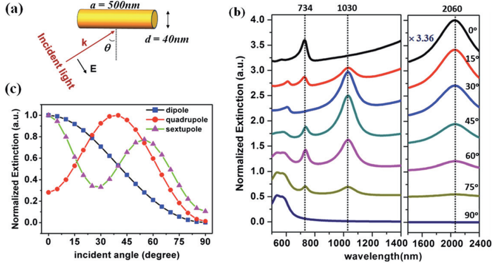
FIGURE 1.41 – Adapté depuis Yong et al. 116 (a) Paramètres utilisés pour la simulation numérique. (b) Simulations des spectres d'extinction du nanobâtonnet pour différents angles \theta . Les valeurs du panneau de gauche sont normalisées par le mode quadripolaire à 1030 nm pour \theta = 45^\circ et le panneau de droite par le mode dipolaire pour \theta = 0^\circ . (c) Évolution de l'extinction des différents modes en fonction de l'angle d'incidence, normalisée par le maximum respectif de chacun des modes.
