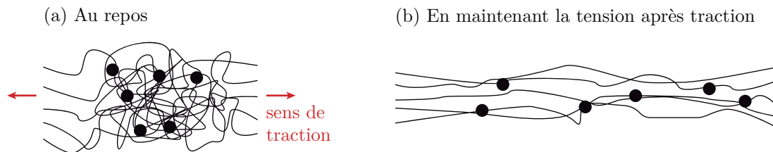
FIGURE 1.2 – (a) Polymère thermodurcissable au repos et (b) durant un essai de traction : les chaînes s'alignent parallèlement à l'axe de traction, impliquant une entropie négative.
