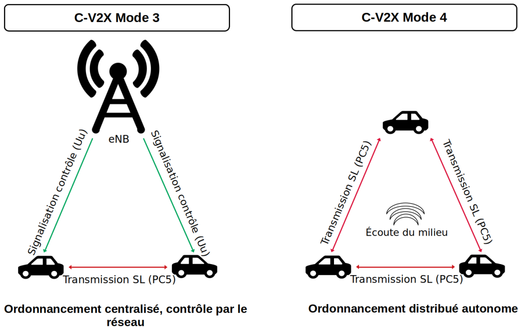
FIGURE 4.3 Modes de communication 3 et 4 du C-V2X.
