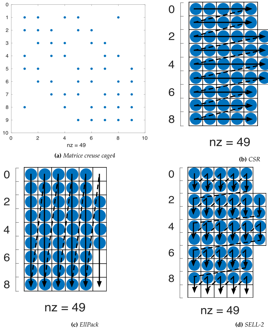
Figure 3.1 – Des exemples de représentation des formats de stockage CSR (3.1b), EIPack (3.1c) et SELL-2 (3.1d) de la matrice creuse cake4 .
